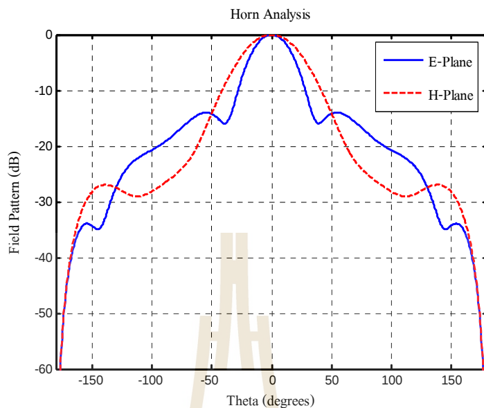
(ข) แบบรูปการแผ่พลังงานในพิกัดสี่เหลี่ยม
