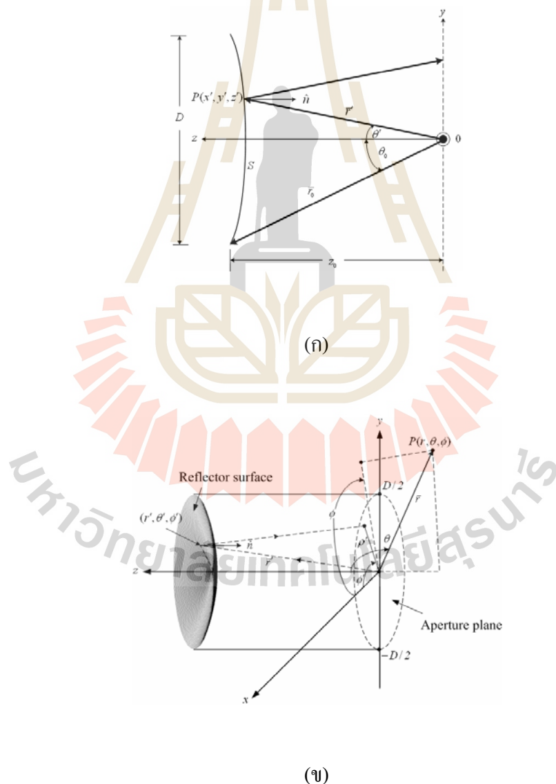
รูปที่ 4.7 เรขาคณิตของสายอากาศตัวสะท้อนในสองมิติและสามมิติ
