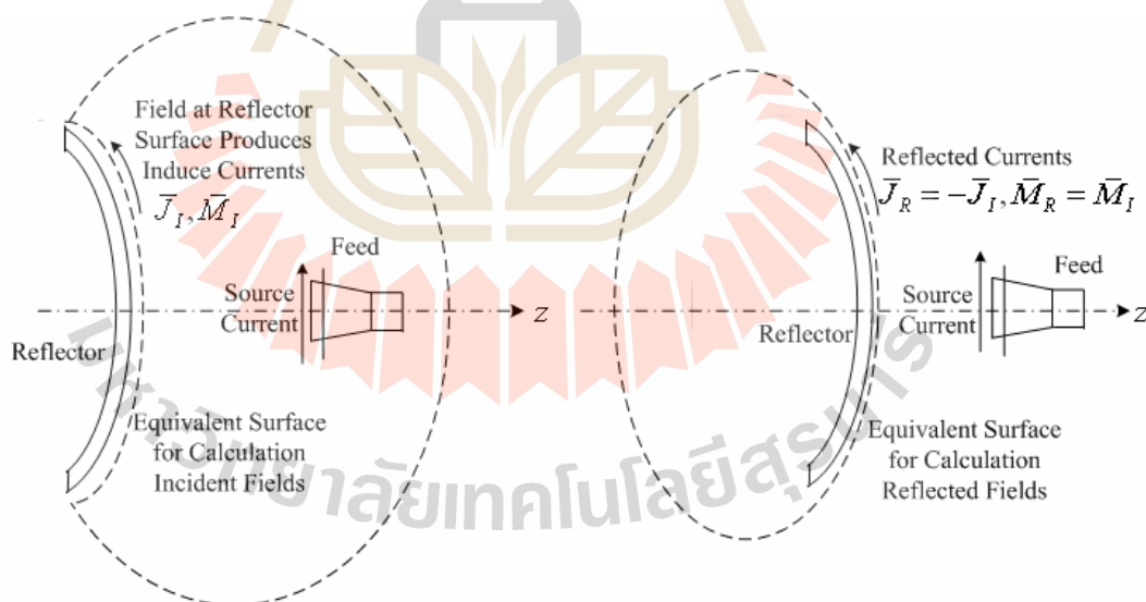
รูปที่ 4.6 พื้นผิวสมมูลเพื่อใช้ในการคำนวณหาสนามที่สะท้อนออกจากตัวสะท้อน
