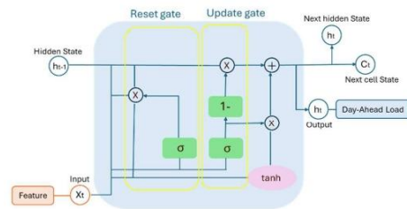
Fig. 3. GRU architecture.
