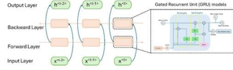
Fig. 4. Bi-GRU architecture.
