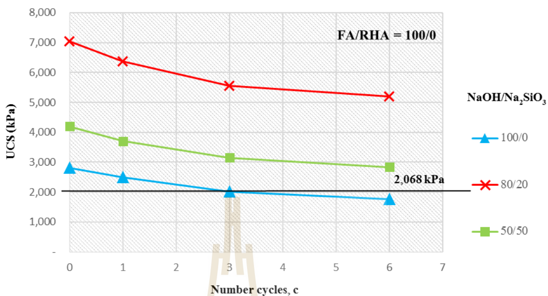
รูปที่ 4.2 ความสัมพันธ์ระหว่างกำลังอัดของมวลรวมผิวทางแอสฟัลต์คอนกรีตที่ ปรับปรุงด้วยจีโอพอลิเมอร์ ผสมเถ้าลอย (FA/RHA = 100/0) กับจำนวนรอบ เปียกสลับแห้ง
