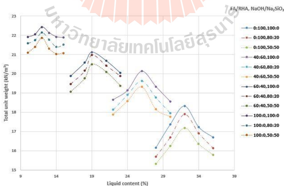
รูปที่ 4.1 ปริมาณสารเชื่อมประสานที่เหมาะสมในแต่ละส่วนผสม
