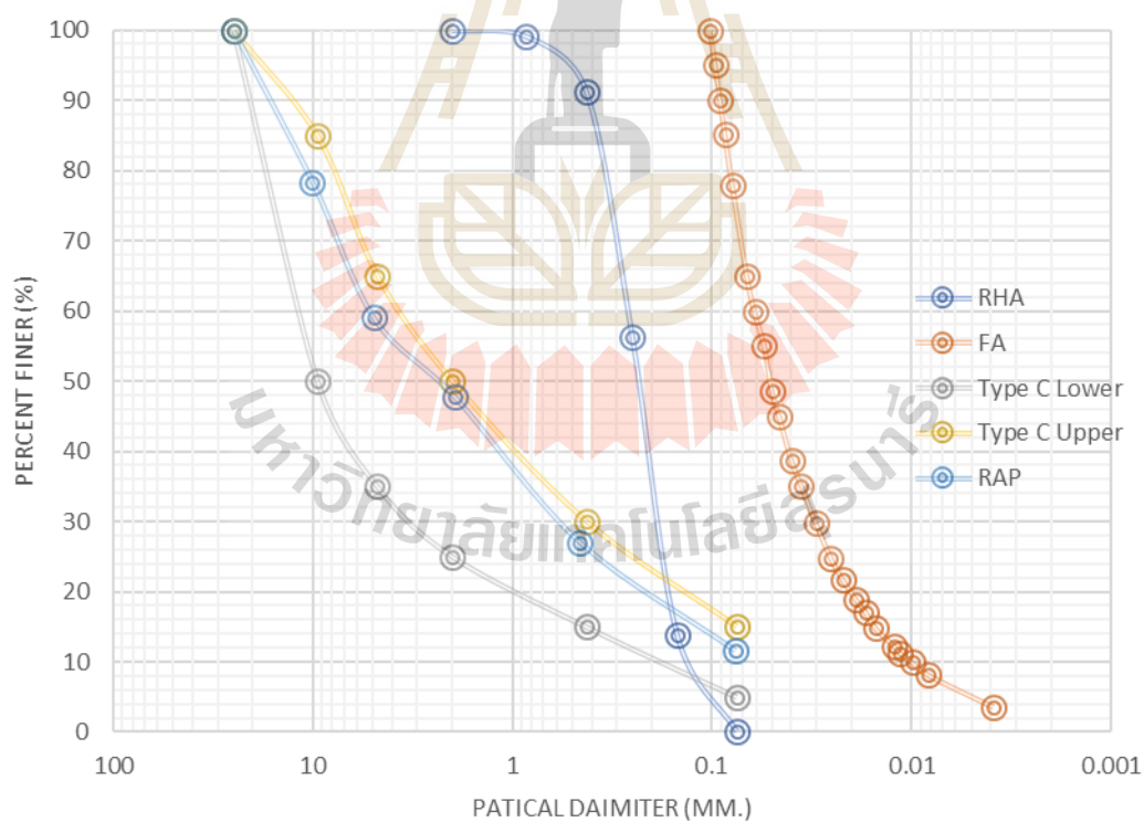
รูปที่ 3.3 การกระจายขนาดผลของมวลรวมผิวทางแอสฟัลต์คอนกรีตไร้ซิลิกา เถ้าลอยและเถ้าแกลบ
