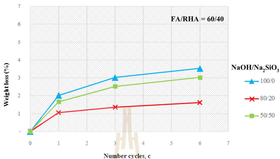
รูปที่ 4.6 ความสัมพันธ์ระหว่างร้อยละการสูญเสียน้ำหนักของมวลรวมผิวทางแอสฟัลต์คอนกรีตที่เสริมด้วยจีโอพอลิเมอร์ ผสมเถ้าลอย/เถ้าแกลบ (FA/RHA = 60/40) กับจำนวนรอบเปียกสลับแห้ง
