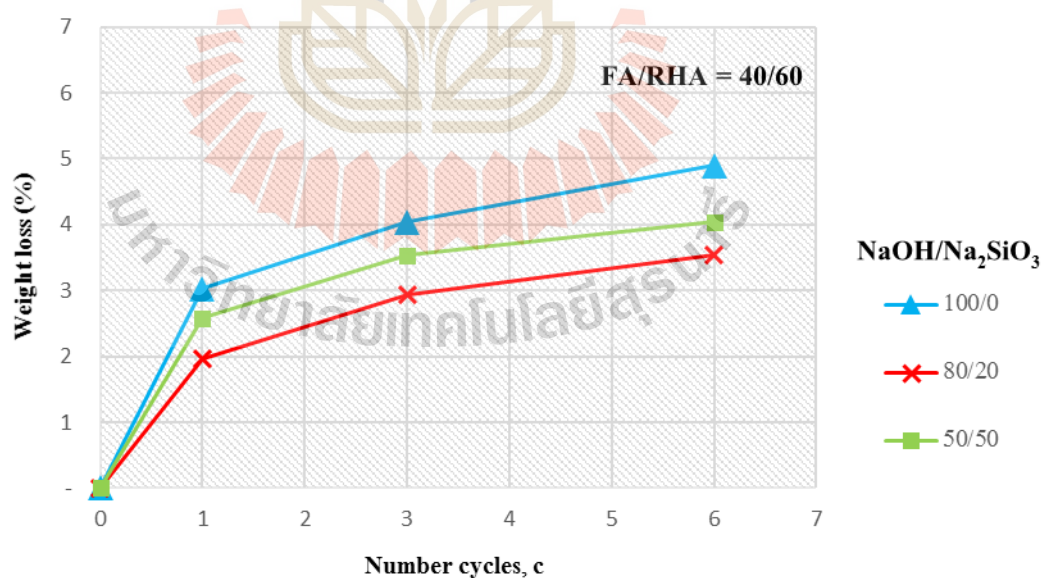
รูปที่ 4.7 ความสัมพันธ์ระหว่างร้อยละการสูญเสียน้ำหนักของมวลรวมผิวทางแอสฟัลต์คอนกรีตที่เสริมด้วยจีโอพอลิเมอร์ ผสมเถ้าลอย/เถ้าแกลบ (FA/RHA = 40/60) กับจำนวนรอบเปียกสลับแห้ง
