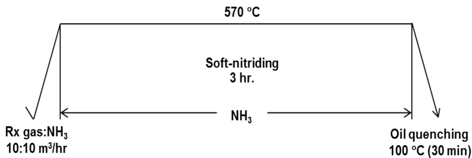
(ก) กระบวนการชุบแข็งแก๊สซอฟต์ไนตรายคิง
