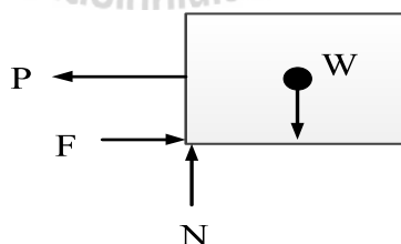
รูปที่ 2.5 แสดงตำแหน่งของแรง N ก่อนที่มวลจะล้มลง
