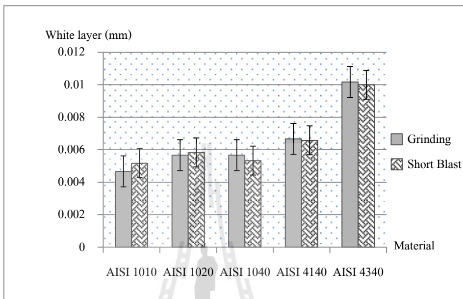
รูปที่ 4.8 กราฟแสดงความสัมพันธ์ของ White layer และประเภทของชั้นทดสอบ กระบวนการแก๊สซัลเฟอร์ในทรายดิ่ง
