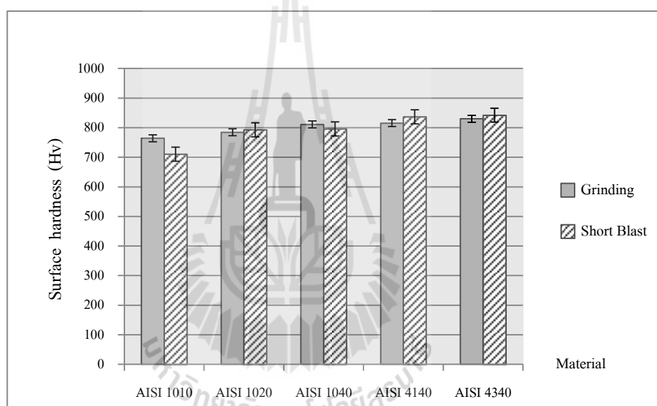
รูปที่ 4.3 แสดงความสัมพันธ์ระหว่าง Surface hardness กับ ประเภทของชั้นทดสอบในกระบวนการแก๊สซอพต์ในทรายดิ่ง
