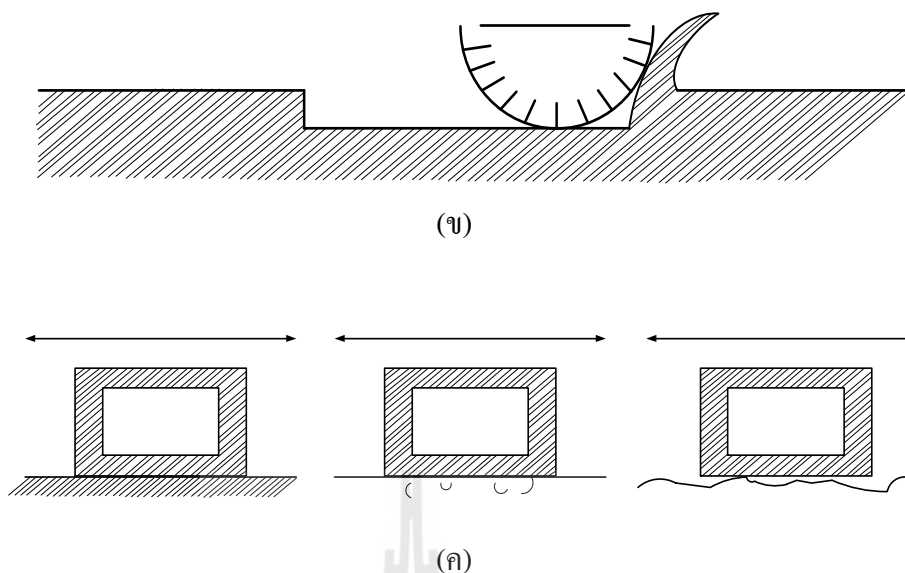
รูปที่ 2.8 การสึกหรอแบบต่าง ๆ (ก) การสึกหรอแบบยึดติด (Adhesive)
