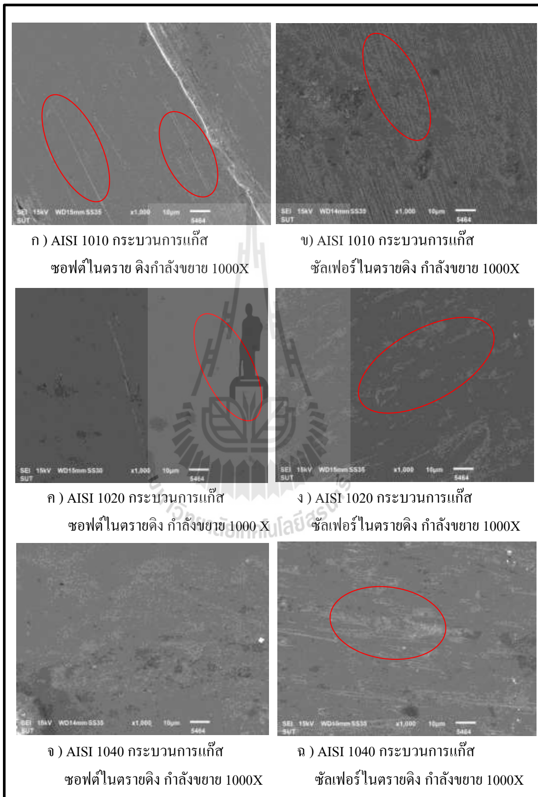
รูปที่ 4.20 แสดงภาพถ่าย SEM พื้นผิวการสึกหรอภายหลังการทดสอบ pin on disc
