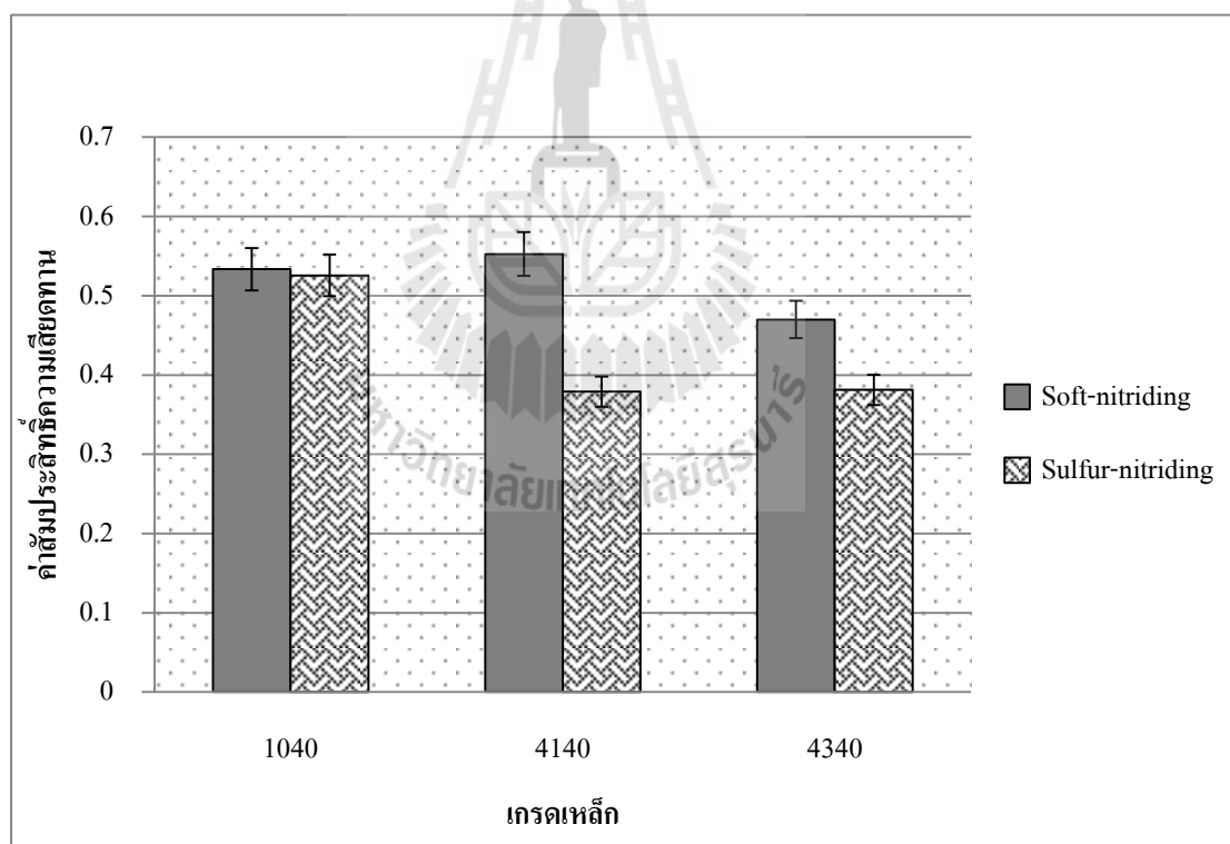
รูปที่ 4.12 กราฟแสดงความสัมพันธ์ระหว่างค่าสัมประสิทธิ์ความเสียหายกับเหล็กกล้าผสมที่นำไปชุบแข็งในกระบวนการต่าง ๆ
