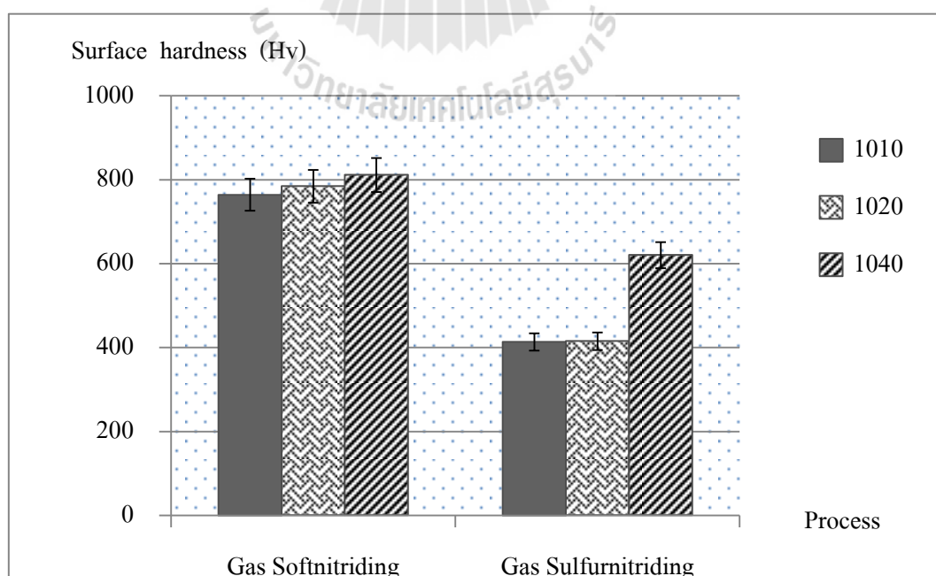
รูปที่ 4.5 กราฟแสดงความสัมพันธ์ของ Surface hardness ในกระบวนการอบชุบต่าง ๆ กลุ่มเหล็กกล้าคาร์บอน
