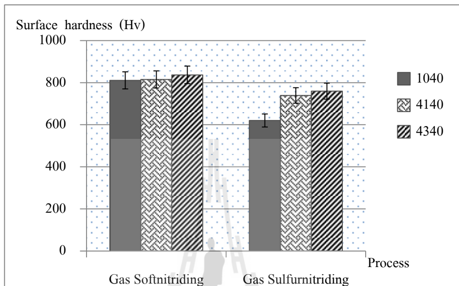
รูปที่ 4.6 กราฟแสดงความสัมพันธ์ของ Surface hardness ที่ผ่านกระบวนการอบชุบต่าง ๆ กลุ่มเหล็กกล้าผสม
