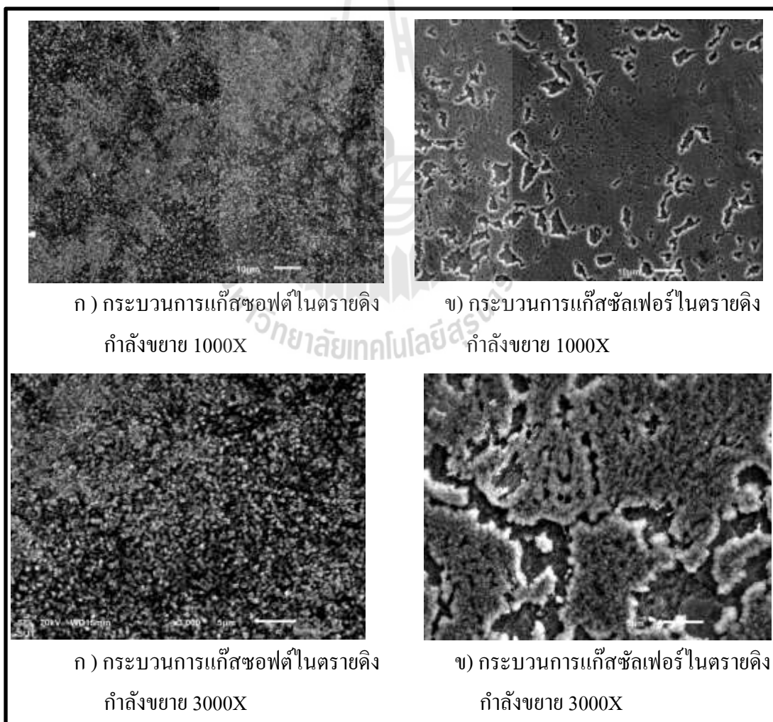
รูปที่ 4.19 แสดงภาพถ่าย SEM (Scanning electron microscope) สภาพผิวหน้าของ หมุดชิ้นทดสอบ
