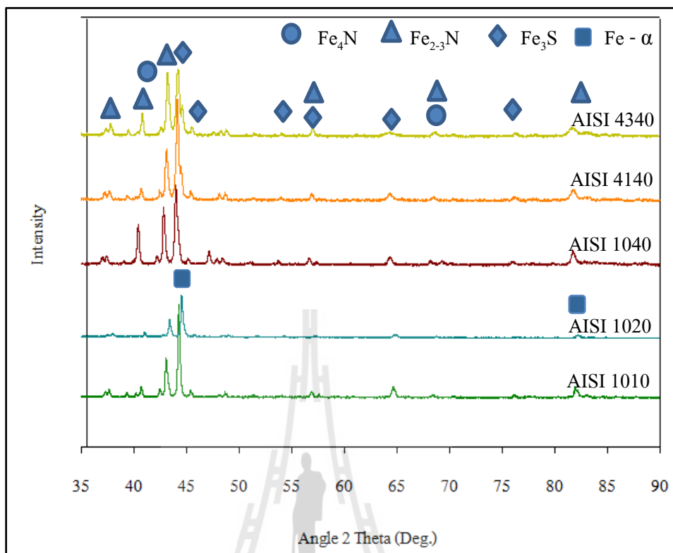
รูปที่ 4.2 กราฟแสดงผลการตรวจสอบการวิเคราะห์ด้วย XRD ด้วยกระบวนการแก๊สซัลเฟอร์ไนโตรเจน
