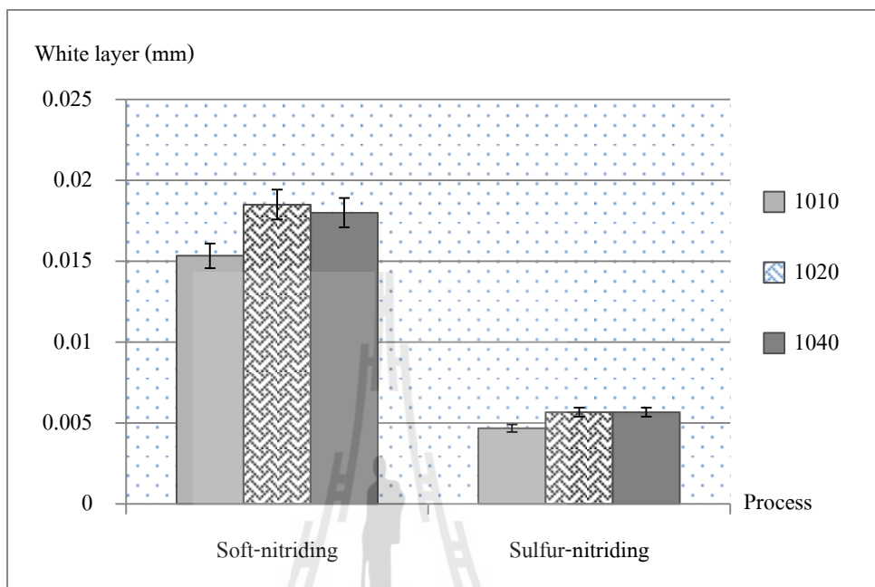
รูปที่ 4.9 กราฟแสดงความสัมพันธ์ของ White layer ที่ผ่านกระบวนการอบชุบต่างๆ เหล็กกล้าคาร์บอน
