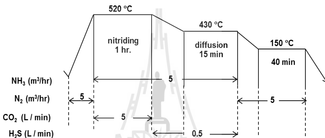
(ก) กระบวนการชุบแข็งแก๊สซอฟต์ไนตรายคิง
