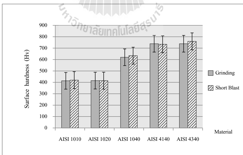
รูปที่ 4.4 แสดงความสัมพันธ์ระหว่าง Surface hardness กับ ประเภทของชั้นทดสอบในกระบวนการแก๊สซัลเฟอร์ในทรายดิ่ง
