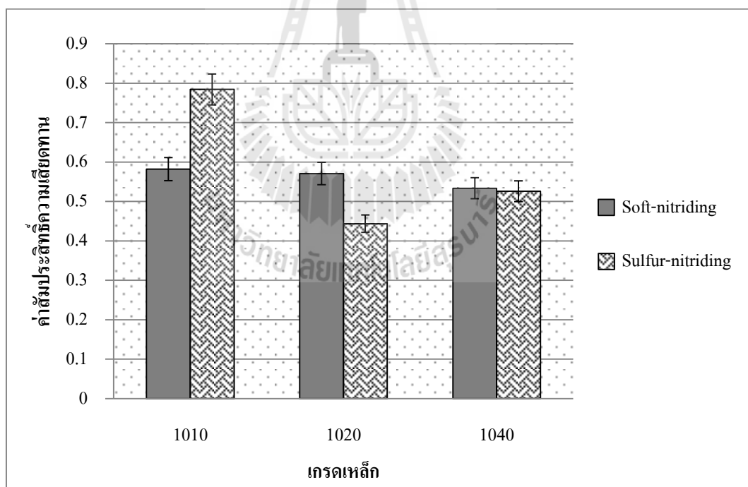
รูปที่ 4.11 กราฟแสดงความสัมพันธ์ระหว่างค่าสัมประสิทธิ์ความเสียหายกับเหล็กกล้าคาร์บอนที่นำไปชุบแข็งในกระบวนการต่าง ๆ
