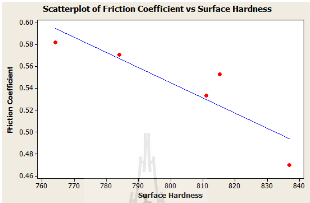
รูปที่ 4.16 ผลการวิเคราะห์ Regression ของค่าสัมประสิทธิ์ความเสียดทาน และค่าความแข็งผิวกระบวนการแก๊สซอฟต์ในทรายดิ่ง
