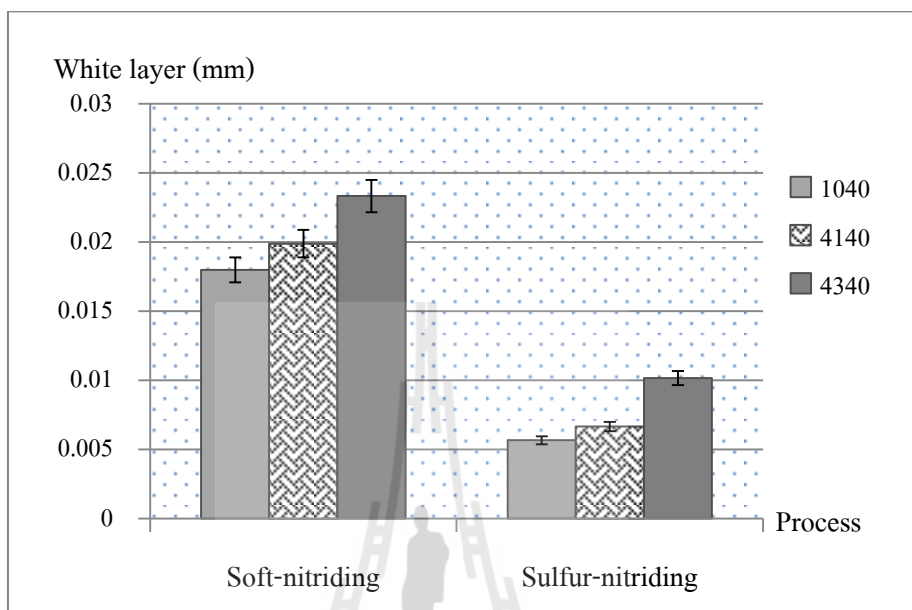
รูปที่ 4.10 กราฟแสดงความสัมพันธ์ของ White layer ที่ผ่านกระบวนการอบชุบต่าง ๆ ในเหล็กกล้าผสม
