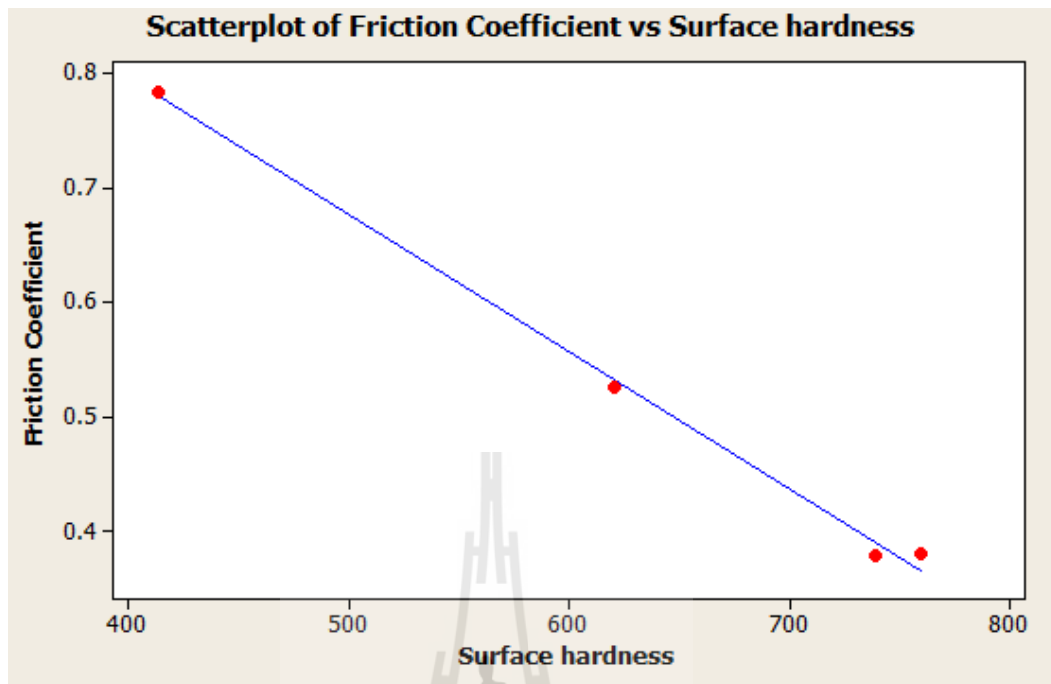
รูปที่ 4.18 ผลการวิเคราะห์ Regression ของค่าสัมประสิทธิ์ความเสียดทาน และค่าความแข็งผิวกระบวนการแก๊สซัลเฟอร์ในทรายดีง
