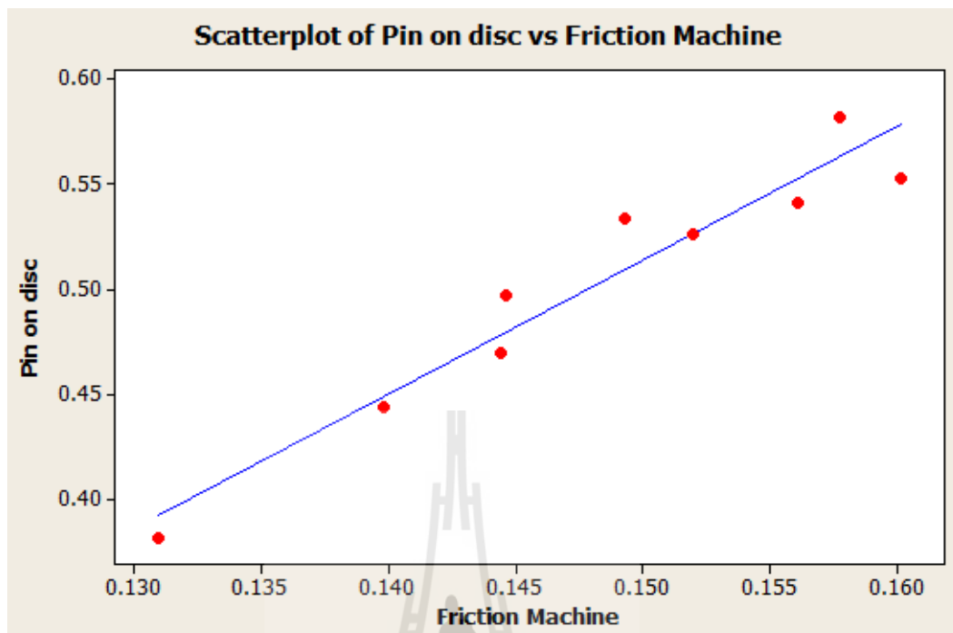
รูปที่ 4.14 กราฟแสดงผลการวิเคราะห์ Correlation และ Regression ของเครื่องทดสอบ Pin on disc และเครื่อง Friction Machine
