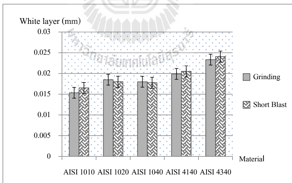
รูปที่ 4.7 กราฟแสดงความสัมพันธ์ของ White layer และประเภทของชั้นทดสอบ กระบวนการแก๊สซัลเฟอร์ไนด์ในทรายดีง
