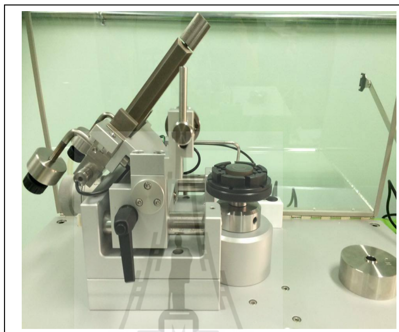
รูปที่ 3.10 เครื่องมือทดสอบ pin on disc (เครื่องธรณศาสตร์)
