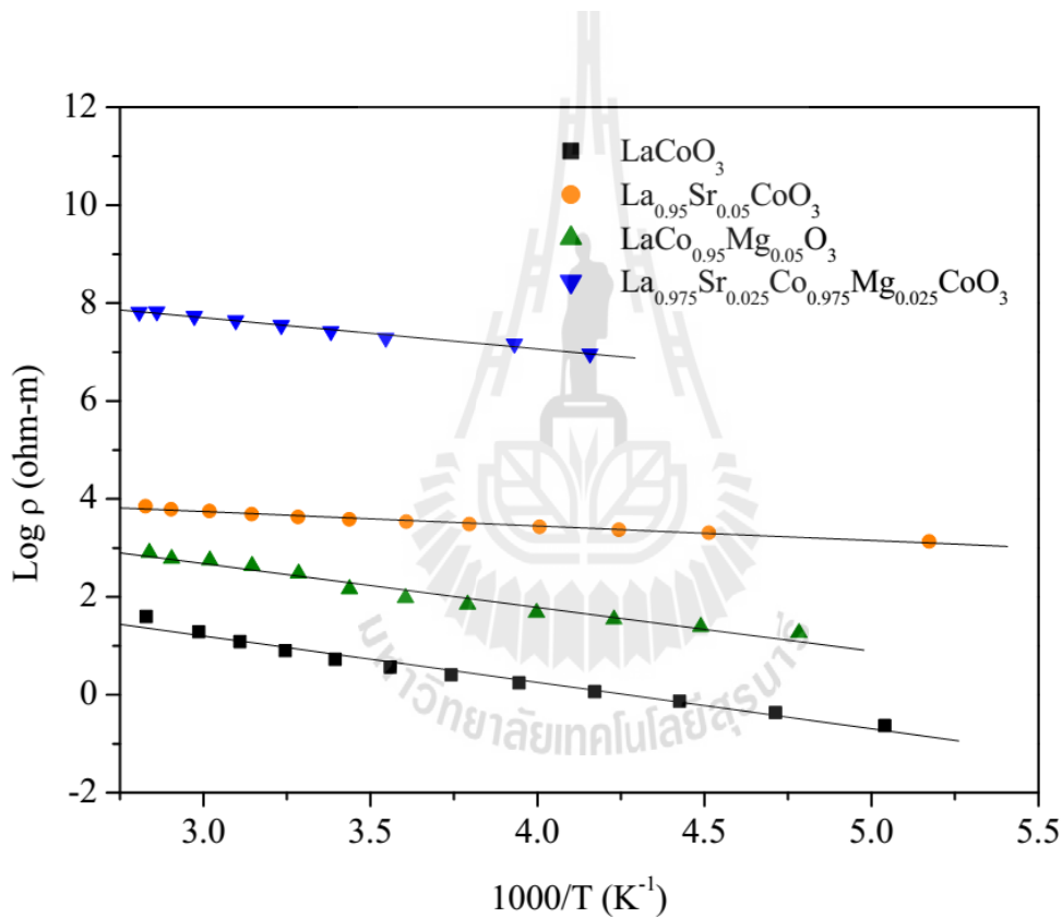
รูป 9 Arrhenius plot ของสารตัวอย่าง
