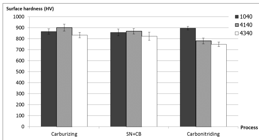
รูปที่ 4.8 แสดงความสัมพันธ์ระหว่าง Surface Hardness กับกระบวนการชุบแข็งผิวในกลุ่มเหล็กกล้าผสม
