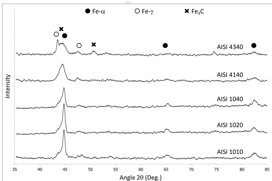
รูปที่ 4.5 แสดงรูปผลการวิเคราะห์ด้วย XRD ในชั้นทดสอบที่กระบวนการร่วมระหว่างแก๊สซอพต์ไนตรายดิงกับแก๊สคาร์บูไรซิง
