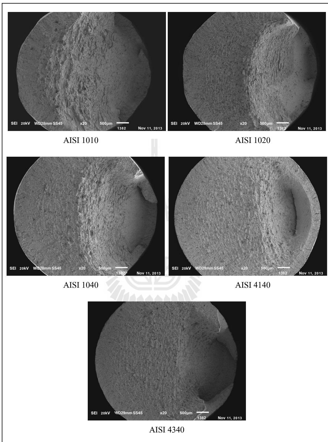
รูปที่ 4.26 แสดงภาพถ่าย SEM บริเวณรอยแตกจากการทดสอบแรงดึงของชิ้นทดสอบเหล็กกล้า ที่ผ่านกระบวนการชุบแข็งผิวด้วยกระบวนการร่วมระหว่างแก๊สคาร์บูไรซิง กับแก๊สซอพต์ไนตรายดิง
