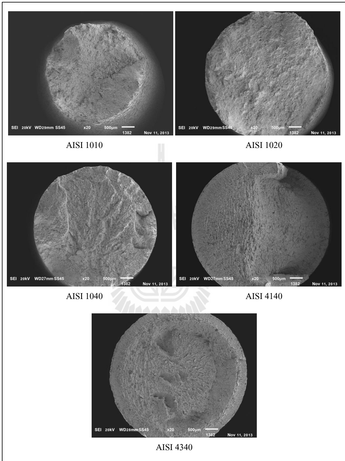
รูปที่ 4.25 แสดงภาพถ่าย SEM บริเวณรอยแตกจากการทดสอบแรงดึงของชิ้นทดสอบเหล็กกล้าที่ผ่านกระบวนการชุบแข็งผิวด้วยแก๊สซอพท์ในทรายดิ่ง
