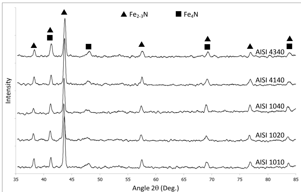
รูปที่ 4.6 แสดงรูปผลการวิเคราะห์ด้วย XRD ในชั้นทดสอบกระบวนการร่วมระหว่างแก๊สคาร์บูไรซิ่งกับแก๊สซอฟต์ไนตรายิ่ง
