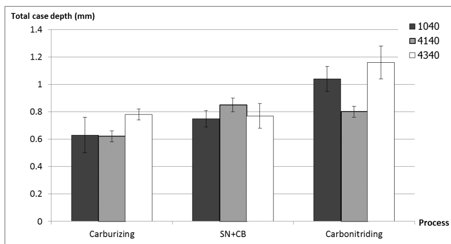
รูปที่ 4.13 แสดงความสัมพันธ์ระหว่าง Total case depth กับกระบวนการชุบแข็งผิวในกลุ่มเหล็กกล้าผสม
