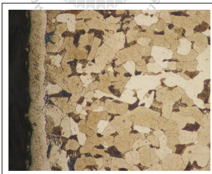
รูปที่ 3.10 แสดงถ่ายภาพขนาดของชั้นผิวขาว ด้วยกล้องจุลทรรศน์แบบออปติคอล กำลังขยาย 400 เท่า
