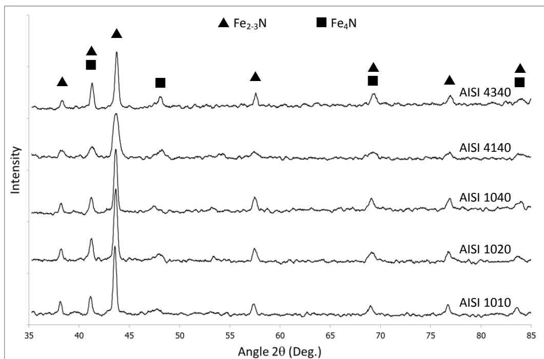
รูปที่ 4.2 แสดงรูปผลการวิเคราะห์ด้วย XRD ในชั้นทดสอบแก๊สซอพต์ในตารางดัง
