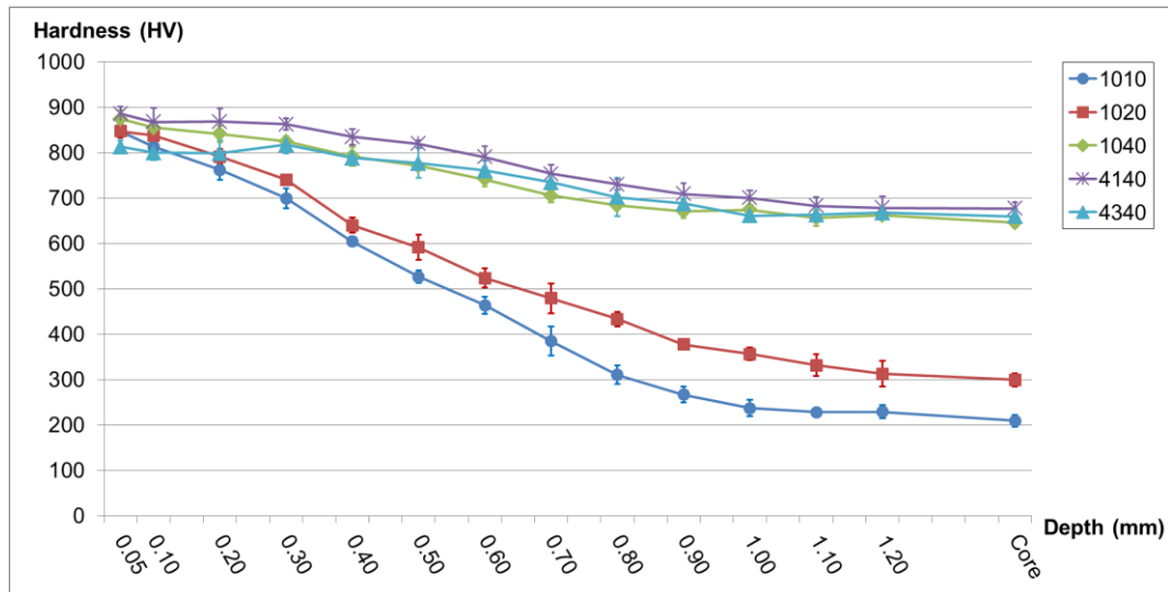
รูปที่ 4.10 แสดงความสัมพันธ์ระหว่าง Hardness กับระยะจากผิวถึงแกนกลางของชิ้นทดสอบ ที่ผ่านกระบวนการร่วมระหว่างแก๊สซอพดีไนตรอยดิงกับแก๊สคาร์บูไรซิง
