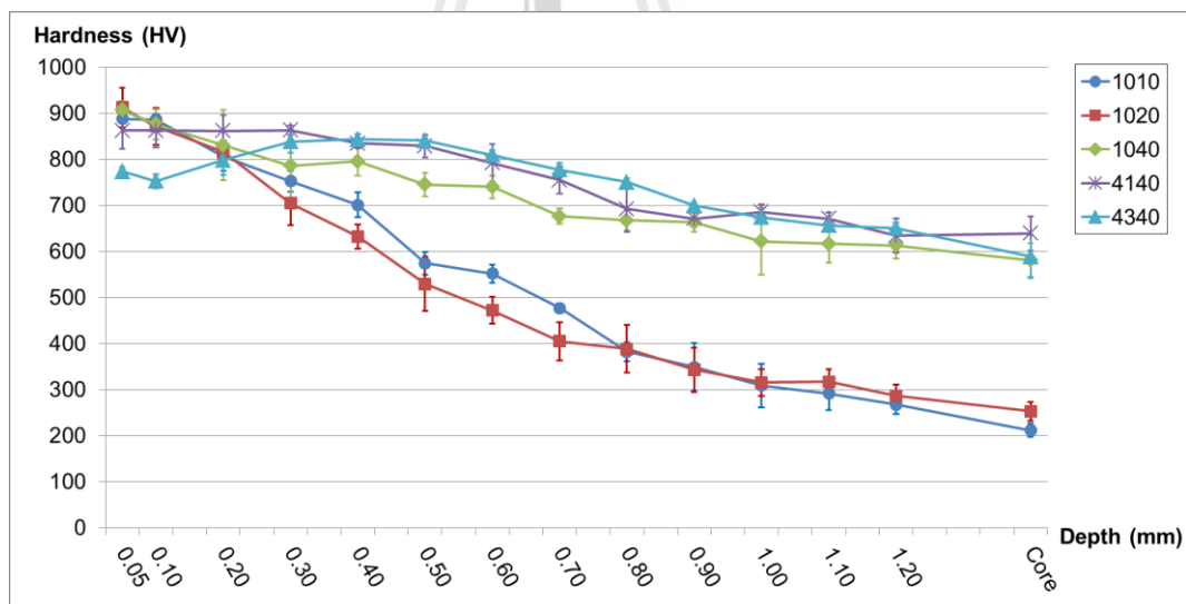
รูปที่ 4.11 แสดงความสัมพันธ์ระหว่าง Hardness กับระยะจากผิวถึงแกนกลางของชิ้นทดสอบ ที่ผ่านการชุบแข็งผิวด้วยแก๊สคาร์โบไนตรอยดิง
