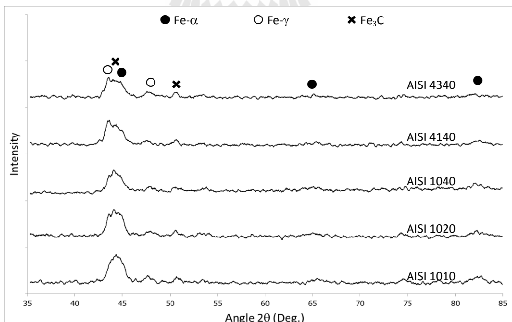
รูปที่ 4.4 แสดงรูปผลการวิเคราะห์ด้วย XRD ในชั้นทดสอบแก๊สคาร์โบไนตรายดิง
