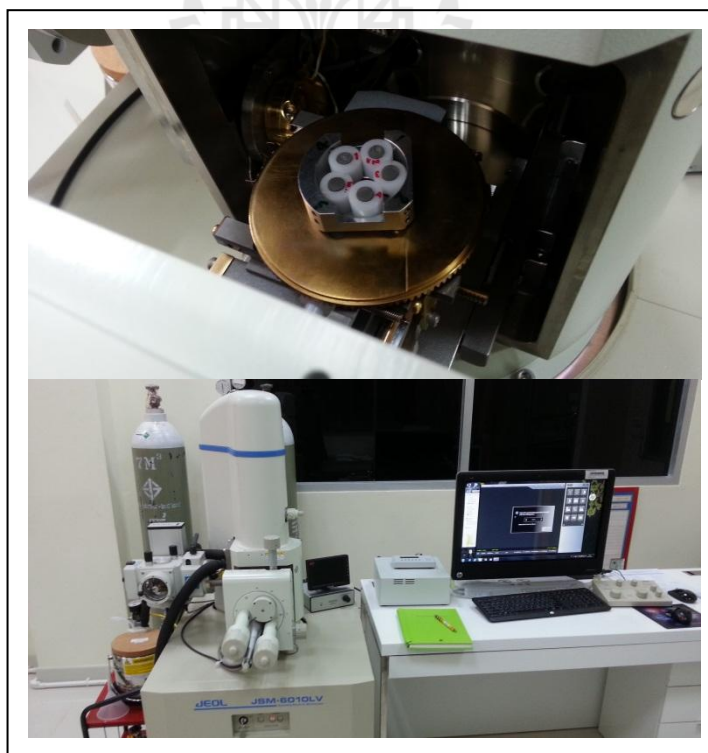
รูปที่ 3.12 แสดงลักษณะการจับยึดชิ้นทดสอบและเครื่อง SEM ที่ใช้ในการทดสอบ
