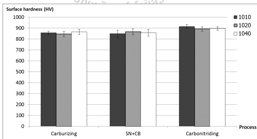
รูปที่ 4.7 แสดงความสัมพันธ์ระหว่าง Surface Hardness กับกระบวนการชุบแข็งผิวในกลุ่มเหล็กกล้าคาร์บอน
