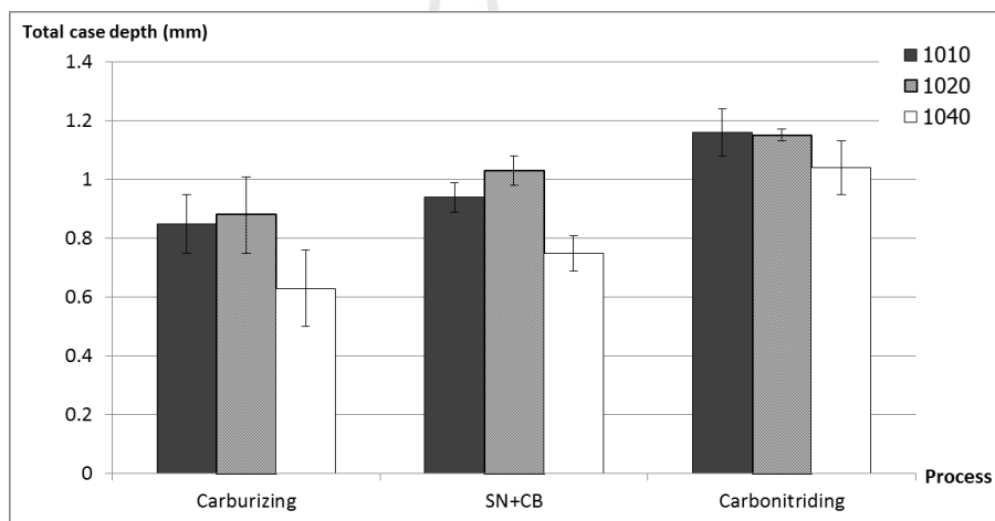
รูปที่ 4.12 แสดงความสัมพันธ์ระหว่าง Total case depth กับกระบวนการชุบแข็งผิวในกลุ่มเหล็กกล้าคาร์บอน
