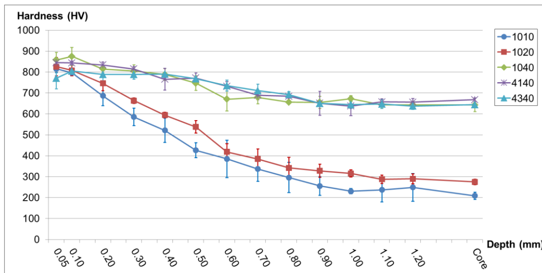
รูปที่ 4.9 แสดงความสัมพันธ์ระหว่าง Hardness กับระยะจากผิวถึงแกนกลางของชิ้นทดสอบ ที่ผ่านการชุบแข็งผิวด้วยแก๊สคาร์บูไรซิง
