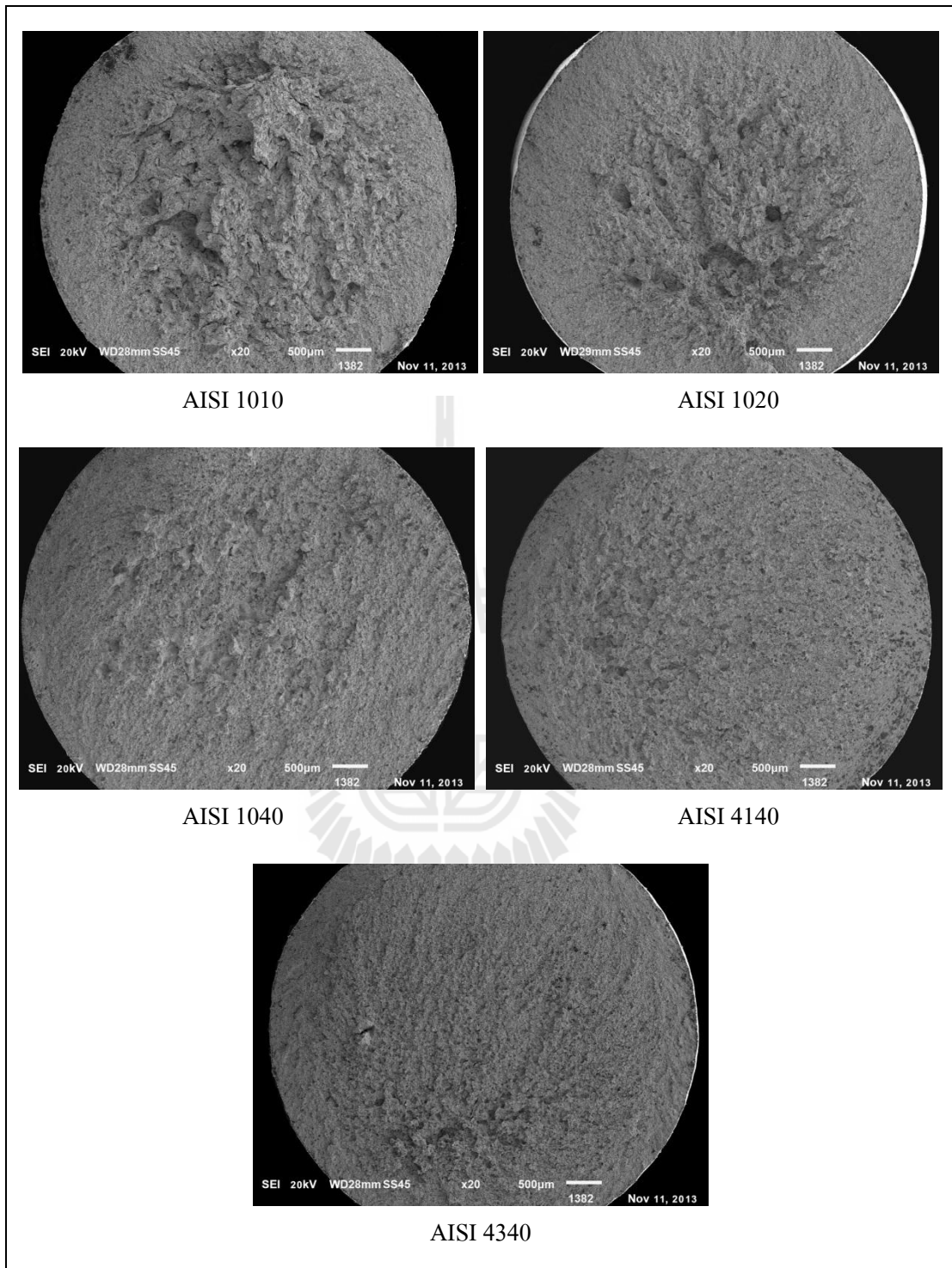
รูปที่ 4.24 แสดงภาพถ่าย SEM บริเวณรอยแตกจากการทดสอบแรงดึงของชิ้นทดสอบเหล็กกล้า ที่ผ่านกระบวนการชุบแข็งผิวด้วยกระบวนการร่วมระหว่างแก๊สซอพตี้ในทรายดิง กับแก๊สคาร์บูไรซิง
