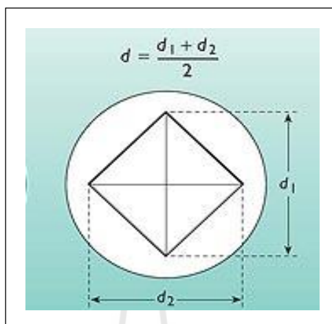
รูปที่ 2.9 แสดงการหาขนาดเส้นทแยงมุมเฉลี่ยในสองแนวซึ่งทำมุมกัน 90 องศา
