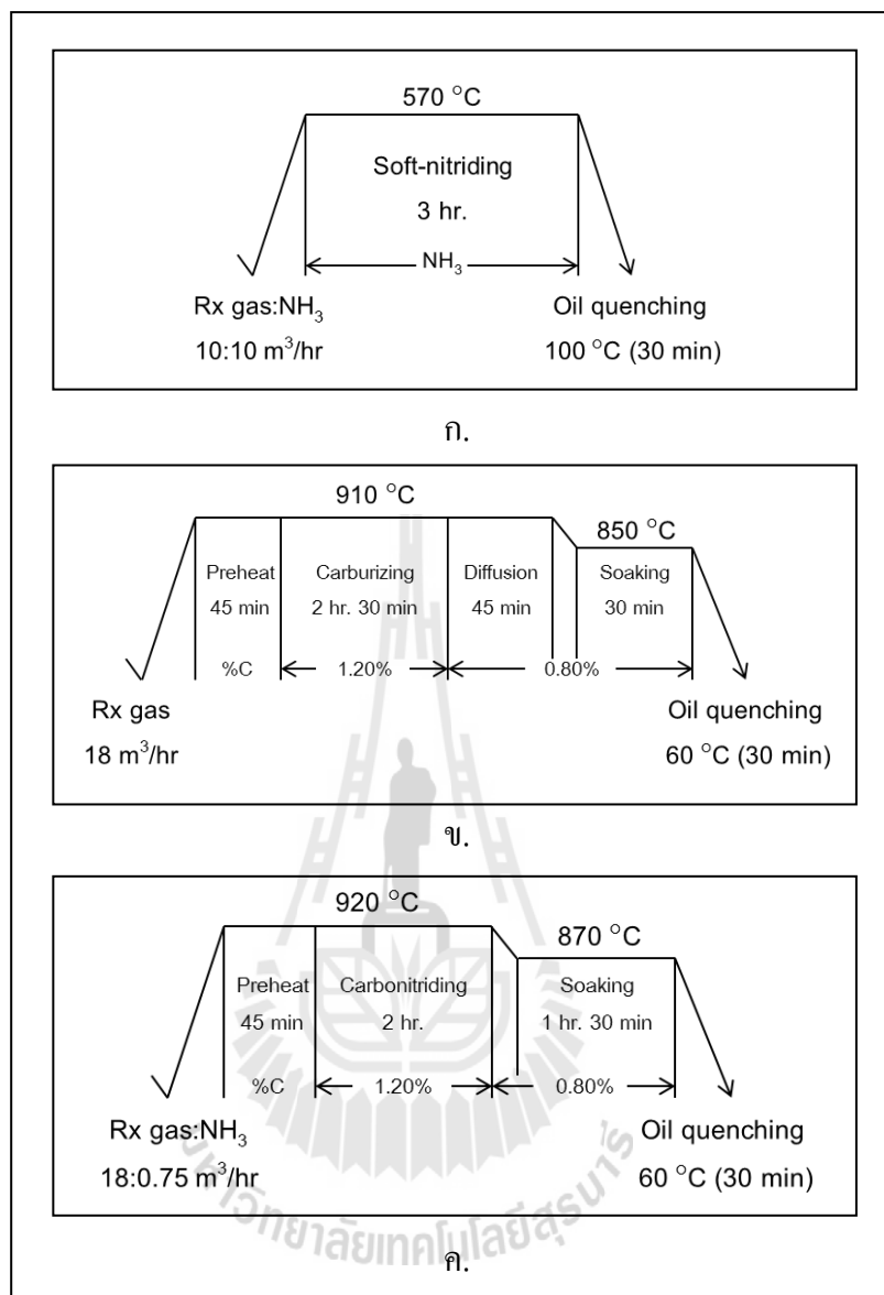
รูปที่ 3.3 แสดงกระบวนการชุบแข็งผิวที่ใช้ในการทดลองทั้งหมด ก. แก๊สซอฟต์ไนตรายคิง (SN) ข. แก๊สคาร์บูไรซิง (CB) และ ค. แก๊สคาร์โบไนตรายคิง (CN)
