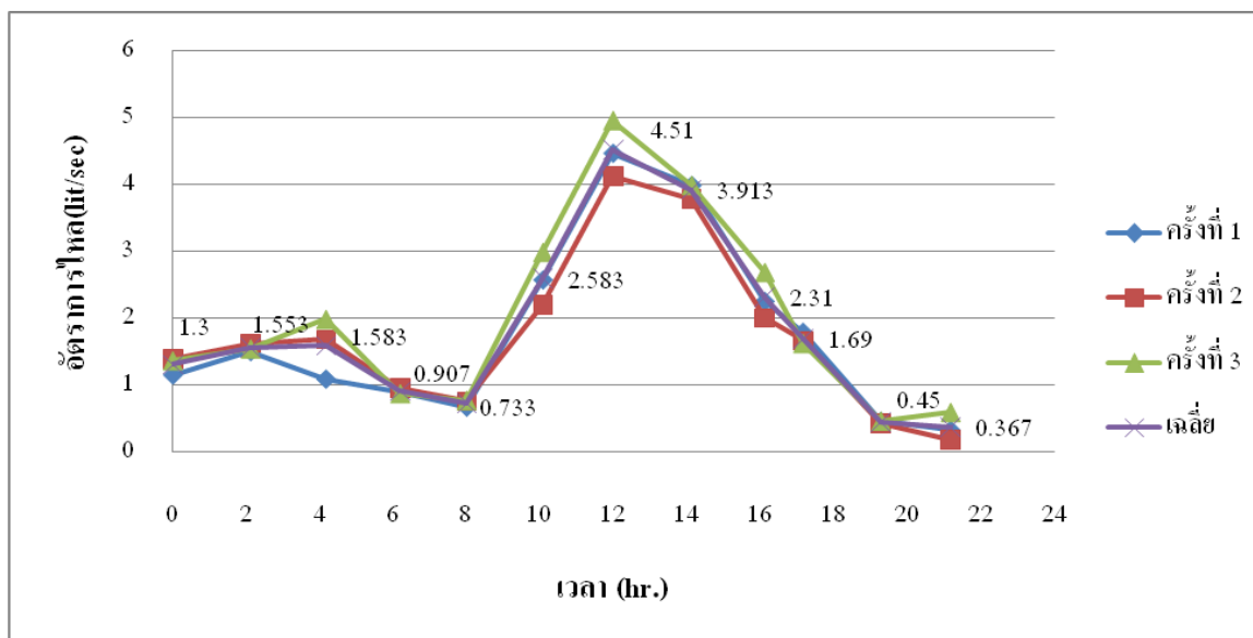
รูปที่ 4.5 กราฟแสดงผลการวัดอัตราการไหลของน้ำเสีย จุดปล่อยน้ำที่ 3
