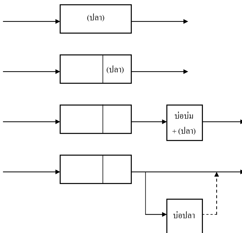
รูปที่ 2.5 แบบการเลี้ยงปลาแบบต่าง ๆ ในระบบบ่อปรับเสถียร (ที่มา Arceivala , S.J. , 1998)
