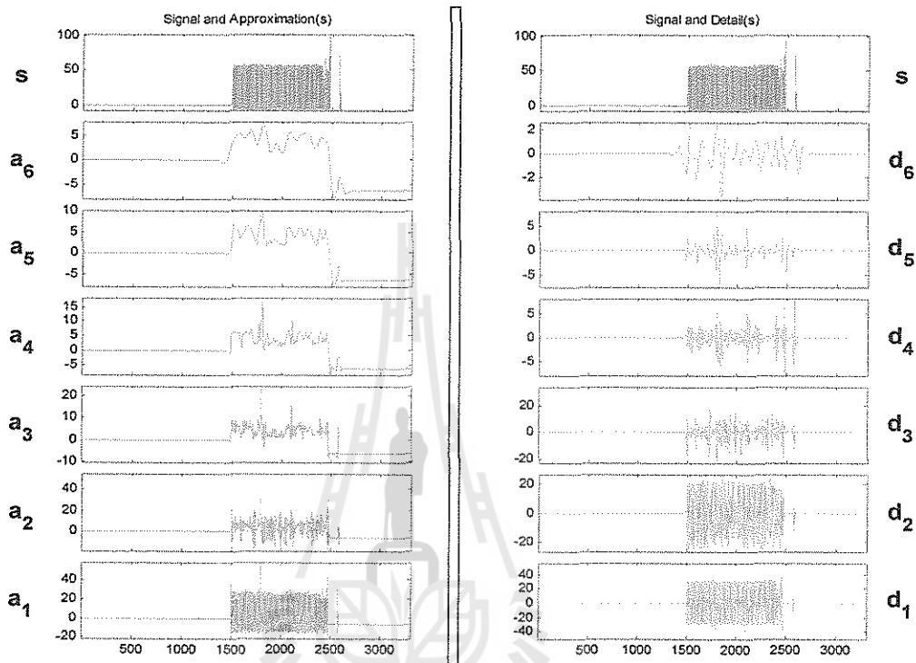
รูปที่ 3.6 สัญญาณ Approximation และสัญญาณ Detail ของ Wavelet DWT ชนิด Db4
