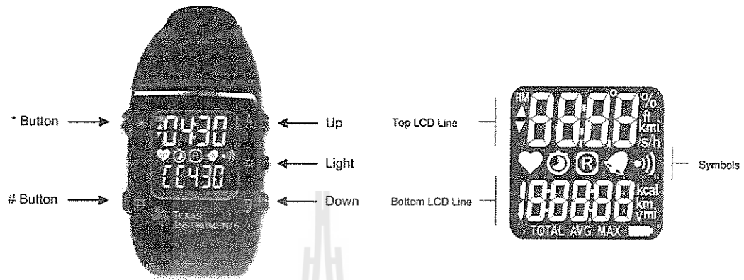
รูปที่ 3.3 eZ430-Chronos Watch
