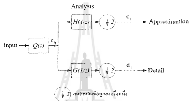
รูปที่ 2.2 การวิเคราะห์สัญญาณด้วยฟังก์ชันเวฟเลต
