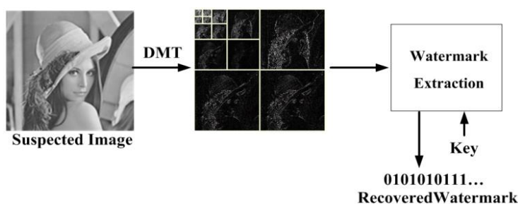
รูปที่ 3.4 การคัดแยกสัญญาณลายน้ำ
