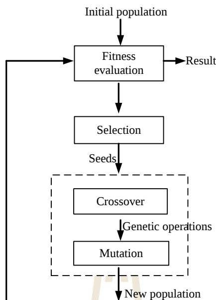
รูปที่ 3.5 แผนภาพการทำออปติไมซ์เซชันด้วย GA
