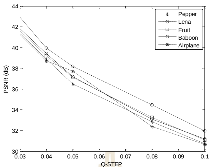
รูปที่ 3.14 เปรียบเทียบค่า PSNR จากการทดสอบที่ค่า Q-step เท่ากับ 0.03, Q-Step-GA, 0.05, 0.08 และ 1.0
