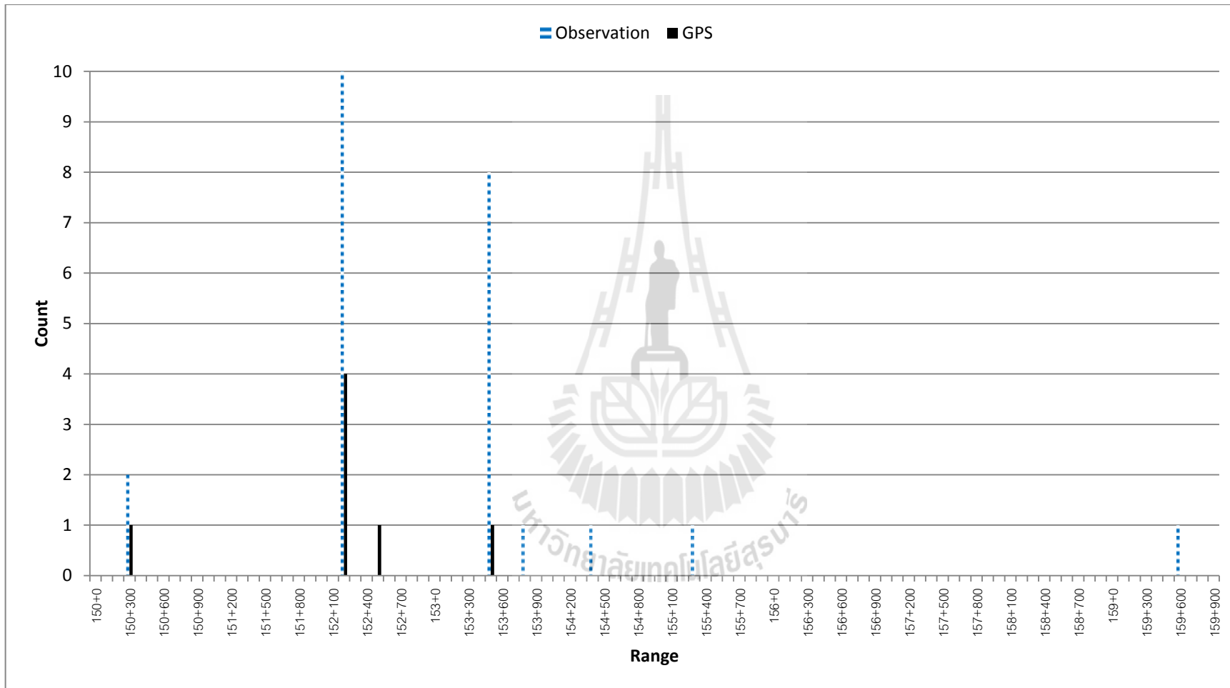
รูปที่ 16 ความถี่ของตำแหน่งคอกขวดที่พบในช่วงกิโลเมตรที่ 150 ถึงกิโลเมตรที่ 159+900
