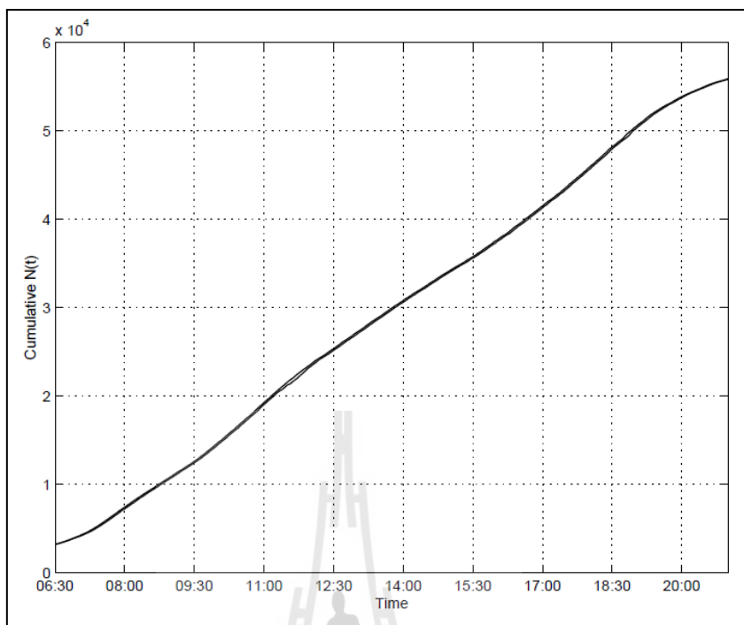
รูปที่ 2.5 แสดงตัวอย่างกราฟความถี่สะสมของตัวตรวจจับ (Detector) 2 ตัวที่อยู่ติดกัน ซึ่งไม่สามารถสังเกตความแตกต่างระหว่างกราฟทั้ง 2 เส้นได้ด้วยตาเปล่า
