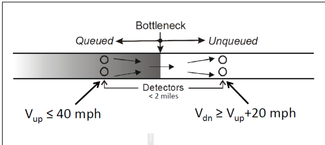
รูปที่ 2.7 แสดงหลักการพิจารณาค่าแห่งคอขวดโดยวิธีการวิเคราะห์ด้วยความเร็วของ Chen.
