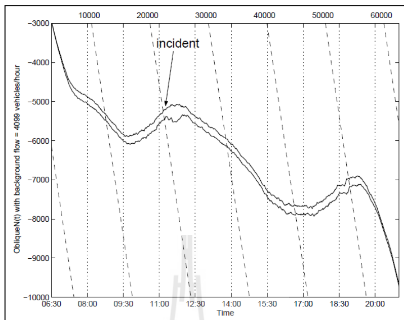
รูปที่ 2.6 แสดงตัวอย่างกราฟความถี่สะสมเชิงเอียงของตัวตรวจจับ (Detector) 2 ตัวที่อยู่ติดกัน ซึ่งสามารถสังเกตความแตกต่างได้อย่างชัดเจนด้วยตาเปล่า
