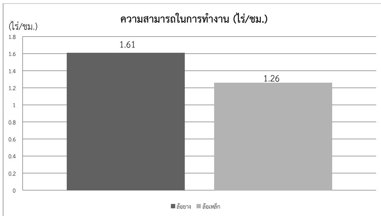
ภาพที่ 9 แสดงการเปรียบเทียบความสามารถในการทำงานของล้อยางและล้อยเหล็ก
