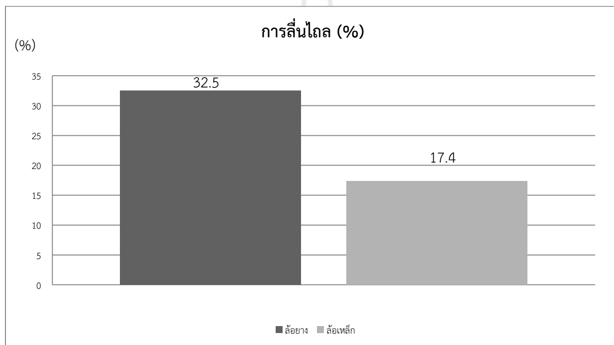
ภาพที่ 7 แสดงการเปรียบเทียบเปอร์เซ็นต์การสิ้นไถของล้อยางและล้อเหล็ก
