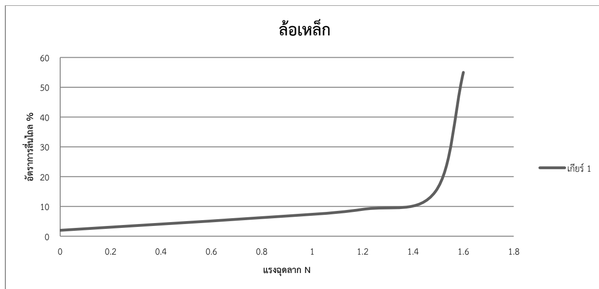
ภาพที่ 16 แสดงการเปรียบเทียบระหว่างอัตราการใช้เชื้อเพลิงและแรงจุดลากของรถไถเดินตามกับล้อยเหล็ก
