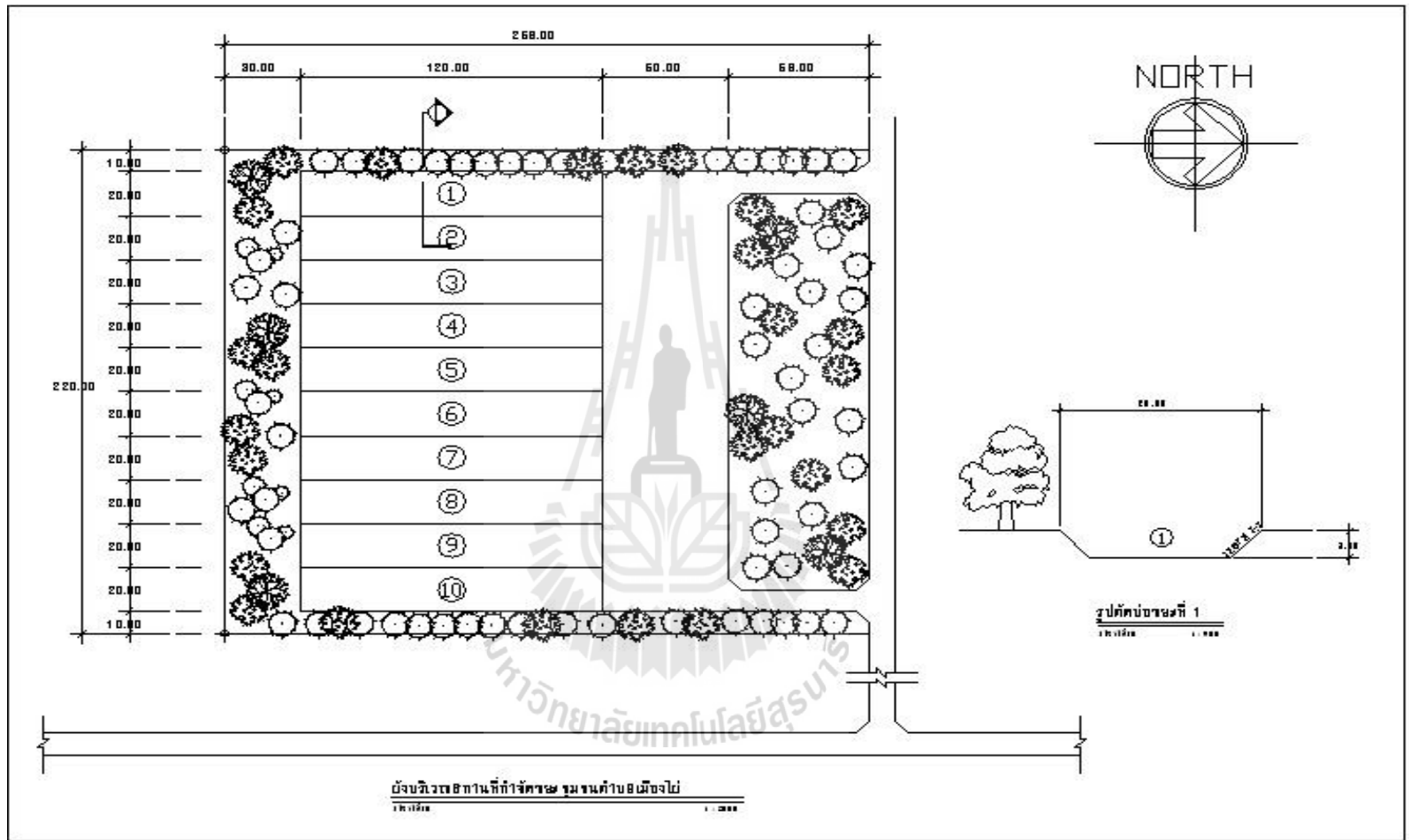
รูปที่ 4.10 แบบก่อสร้างบ่อขยะชุมชนตำบลเมืองไผ่
