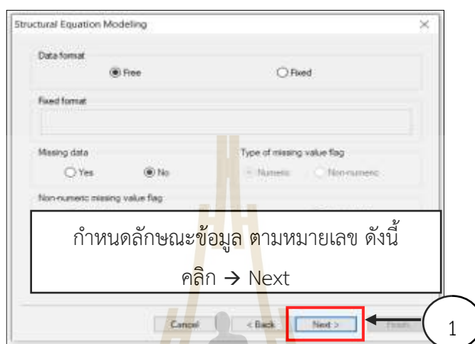
รูปที่ 3.11 การกำหนดลักษณะข้อมูลของตัวแปรในไฟล์ข้อมูลเพื่อวิเคราะห์ CFA
