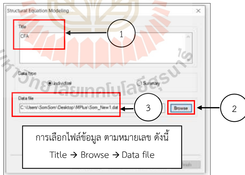
รูปที่ 3.10 การเลือกไฟล์ข้อมูลข้อมูลวิเคราะห์ CFA
