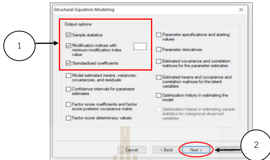
รูปที่ 3.16 การกำหนดรายละเอียดของผลการวิเคราะห์ CFA ใน Printout
