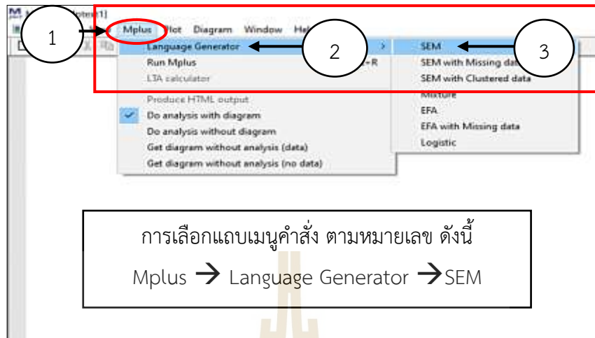
รูปที่ 3.9 การเลือกแถบเมนูคำสั่งการวิเคราะห์ข้อมูล CFA
