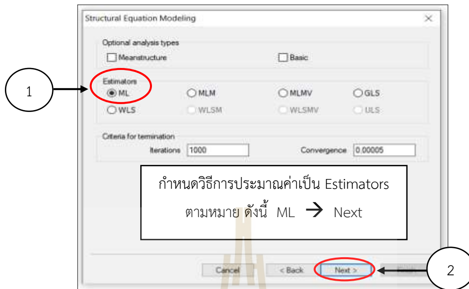
รูปที่ 3.15 การกำหนดวิธีการประมาณค่าพารามิเตอร์สำหรับการวิเคราะห์ CFA
