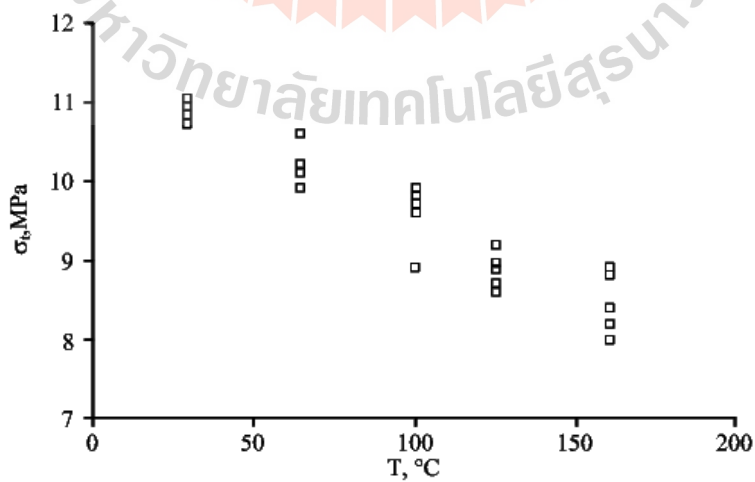
รูปที่ 2.6 ค่ากำลังรับแรงดึงแบบบราซิชของหินแกรนิตภายใต้การผันแปรอุณหภูมิ (Dwivedi et al., 2008)
