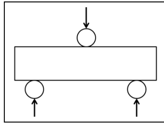
รูปที่ 3.14 การทดสอบแบบจุดรองรับสามจุด
