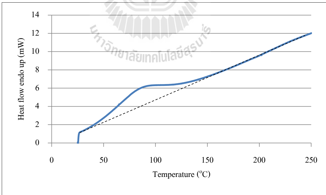
รูปที่ 4.9 กราฟ DSC ของวัสดุที่ขึ้นรูปด้วยการอัดร้อน
