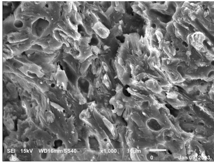
รูปที่ 4.11 วัสดุที่ผสมเศษเมลามีน 0%
