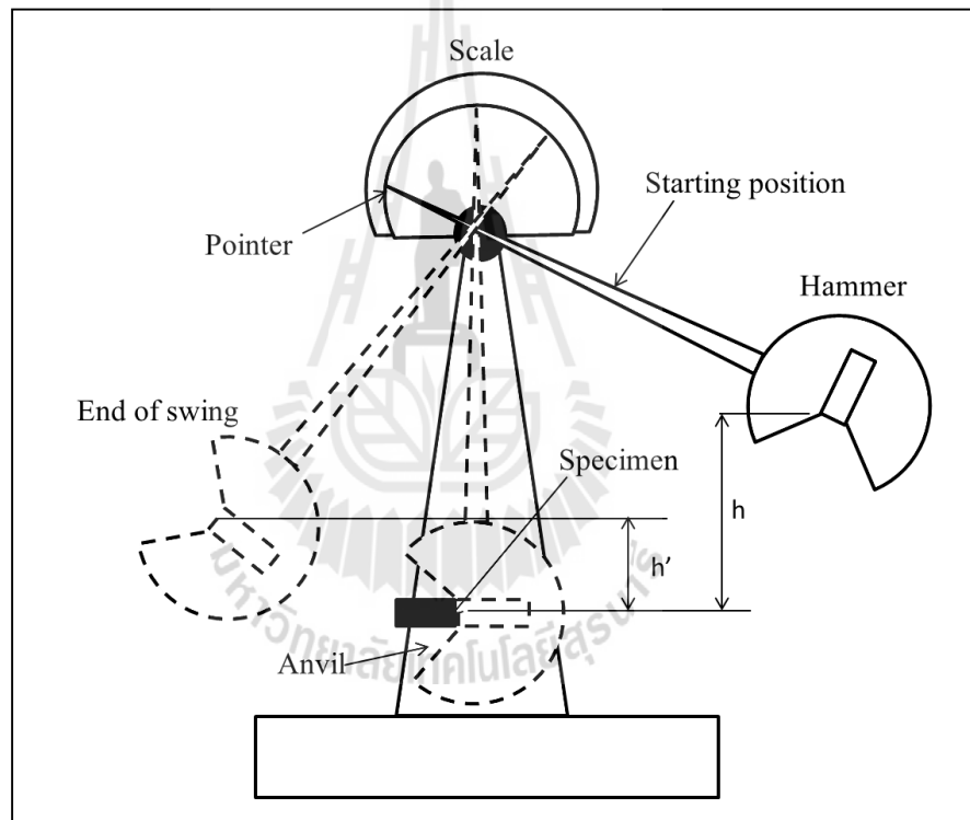
รูปที่ 2.7 ลักษณะการทำงานของเครื่องทดสอบแรงกระแทก
