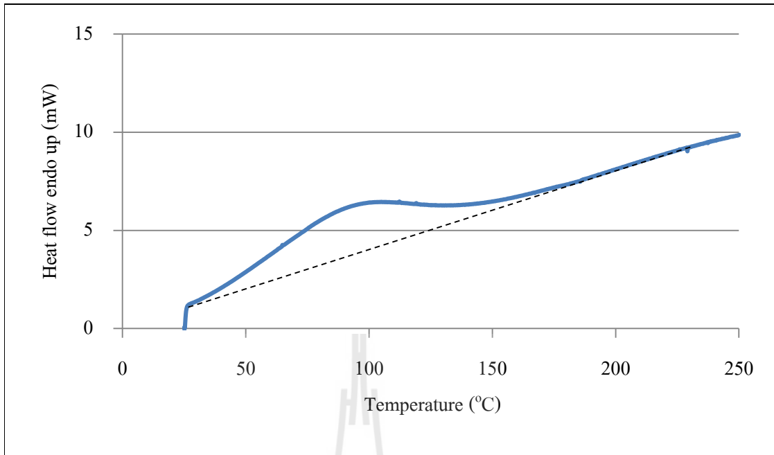
รูปที่ 4.10 กราฟ DSC ของวัสดุที่ขึ้นรูปด้วยการอัดเย็น
