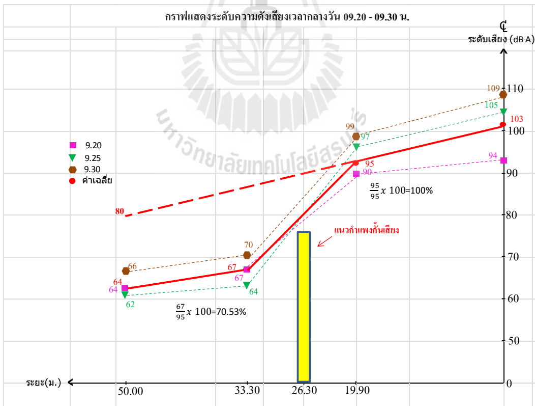
รูปที่ 4.6 กราฟแสดงระดับความดังเสียง เวลา 09.20-09.30 น
