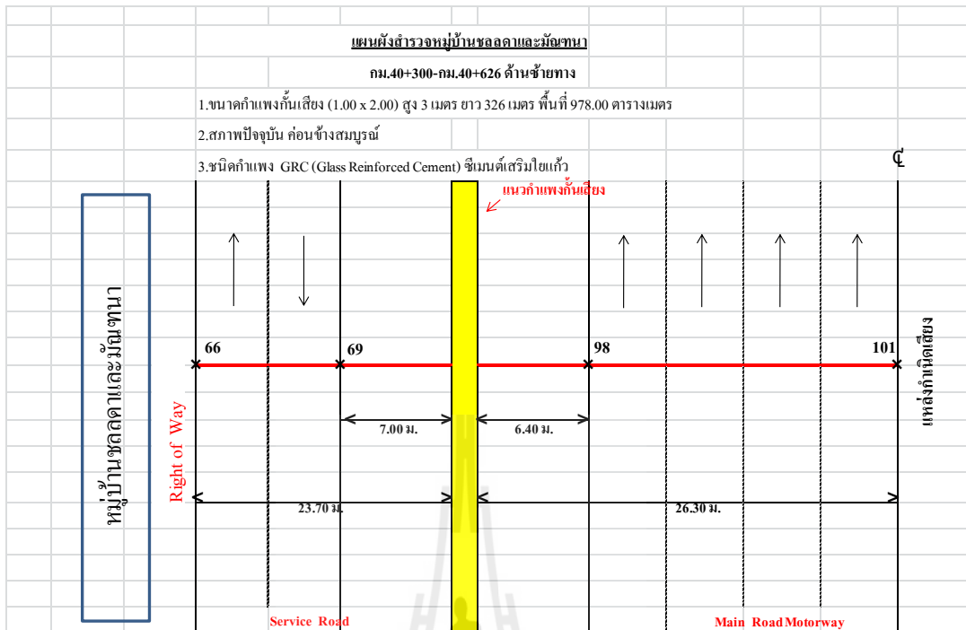
รูปที่ 4.7 แผนผังสำรวจหมู่บ้านชลคาและมัทนา
