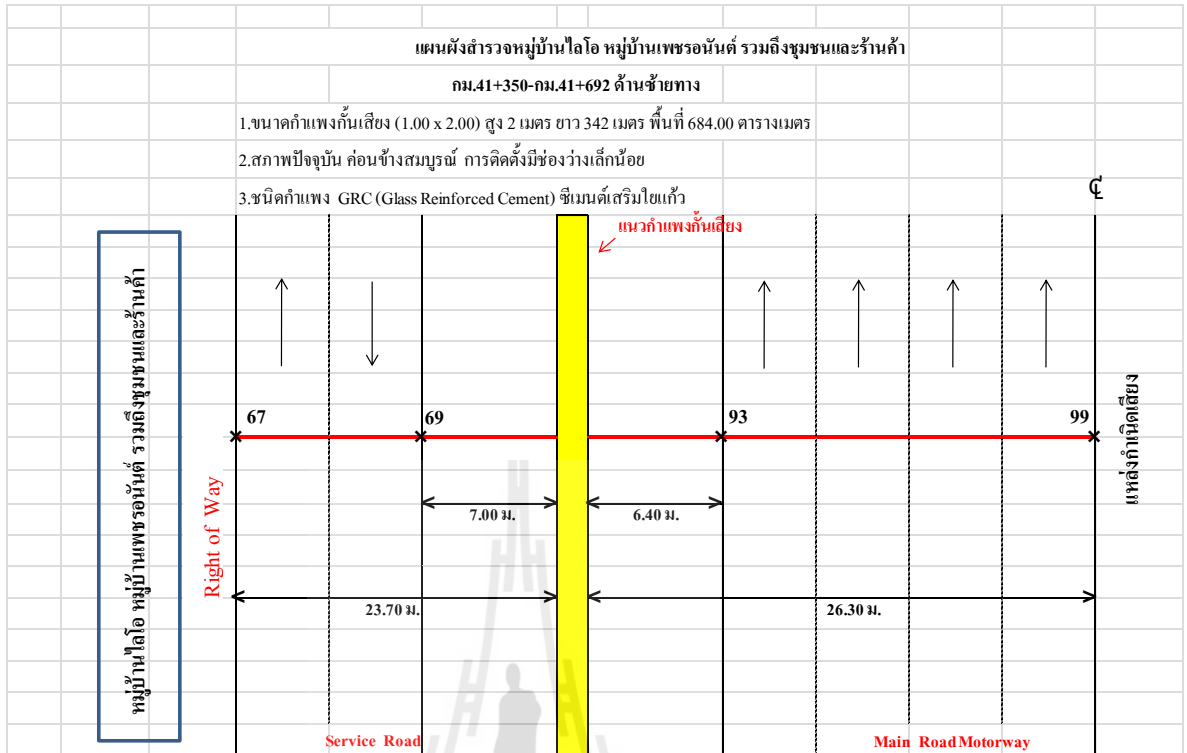
รูปที่ 4.9 แผนผังสำรวจหมู่บ้านไลโอ หมู่บ้านเพชรอนันต์ รวมถึงชุมชนและร้านค้า
