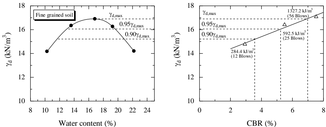
รูปที่ 4.3 ความสัมพันธ์ค่าความแน่นแห้งและค่า ร้อยละCBR ที่พลังงานการบดอัดที่แตกต่างกันของดินเม็ดละเอียด
