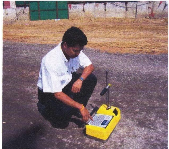
รูปที่ 2.49 การกดแท่งรังสีให้เลื่อนลงไปในรูเจาะให้ลึกตามที่ต้องการ โดยคลายล้อคกลไกที่แขนจับ หลังจากนั้นกดปุ่มคำสั่งให้เครื่องทำงาน
