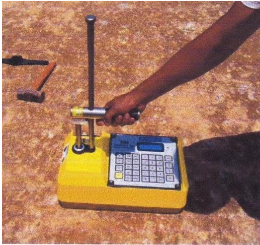
รูปที่ 2.49 การกดแท่งรังสีให้เลื่อนลงไปในรูเจาะให้ลึกตามที่ต้องการ โดยคลายล้อคกลไกที่แขนจับ หลังจากนั้นกดปุ่มคำสั่งให้เครื่องทำงาน
