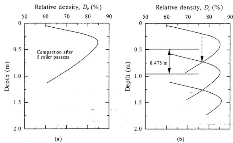
รูปที่ 2.36 การประมาณความหนาแน่นของระดับชั้นของดินสำหรับความหนาแน่นสัมพัทธ์ 75% กับจำนวนรอบของรถบดอัดที่วิ่งผ่านเท่ากับ 5 รอบ
