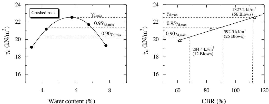
รูปที่ 4.5 ความสัมพันธ์ค่าความแน่นแห้งและค่า ร้อยละ CBR ที่พลังงานการบดอัดที่ต่างกันของหินคลุก
