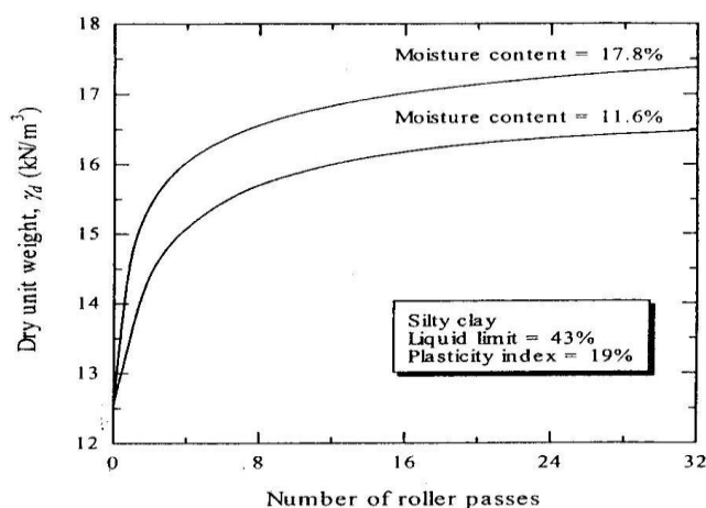
รูปที่ 2.35 a) ความสัมพันธ์ระหว่างความหนาแน่นแห้งและจำนวนรอบของรถดัดที่วิ่งผ่าน (Johnson and Sallberg, 1960)
