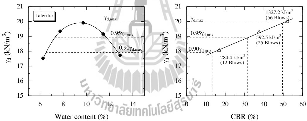
รูปที่ 4.4 ความสัมพันธ์ค่าความแน่นแห้งและค่า ร้อยละCBR ที่พลังงานการบดอัดที่แตกต่างกันของดินลูกรัง
