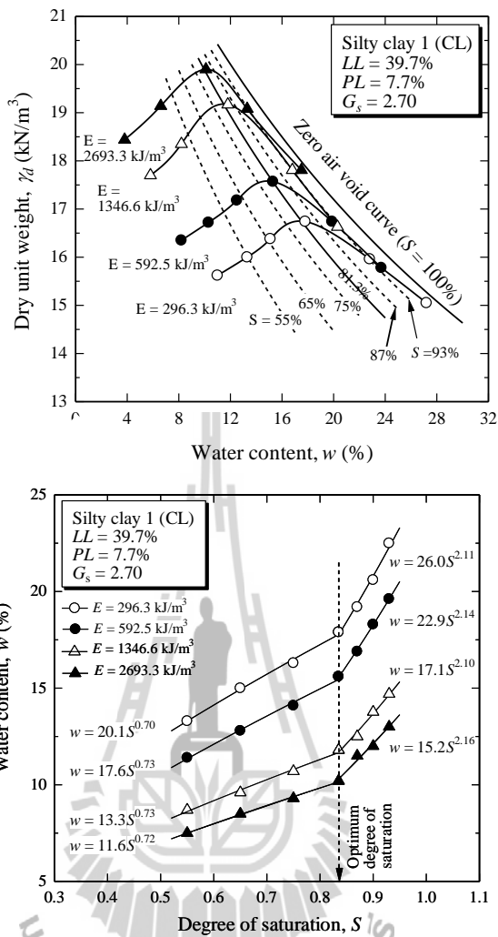
รูปที่ 2.18 (a) กราฟการบดอัด (b) ความสัมพันธ์ระหว่างปริมาณความชื้นและระดับความอิ่มตัว ด้วยน้ำของดินเหนียวปนดินตะกอน (Horpibulsuk et al., 2008a)
