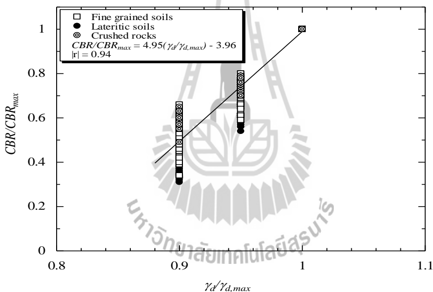
รูปที่ 4.6 กราฟความสัมพันธ์ระหว่างค่า CBR/CBR_{max} และค่า \gamma_d/\gamma_{d,max}
