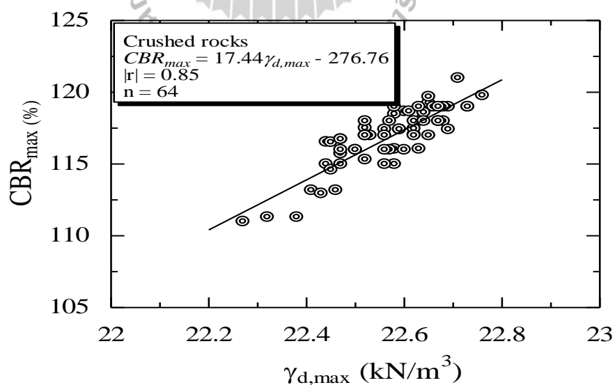
รูปที่ 4.9 กราฟความสัมพันธ์ระหว่างค่าร้อยละ CBR และค่าความแน่นแห้งสูงสุด ( \gamma_d ) Modified Proctor (หินคลุก)
