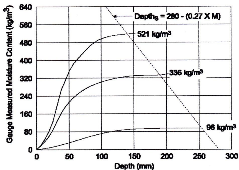
รูปที่ 2.42 กราฟค่าความหนาที่เหมาะสมในการวัดค่าความชื้นในสนามในหน่วย \text{kg/m}^3 top layer effect
