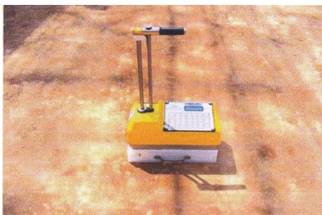
รูปที่ 2.47 การนำเครื่องทดสอบวางบนแผ่นบอลลักราดินเพื่อทำ Standard count
