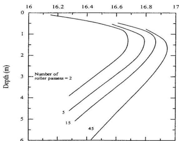
รูปที่ 2.35 b) ความสัมพันธ์ระหว่างหน่วยน้ำหนักแห้งกับจำนวนรอบที่รถดัดวิ่งผ่าน (D'Appolonia et al., 1969)
