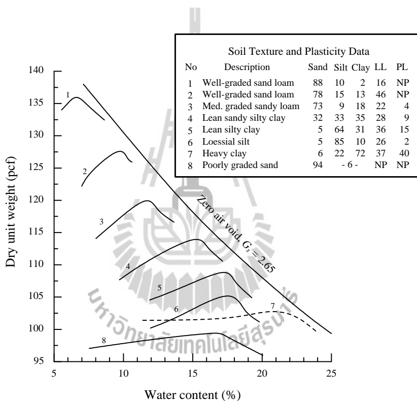
รูปที่ 2.10 อิทธิพลของชนิดดินต่อการบดอัดแบบมาตรฐาน (Johnson and Sallberg, 1960)
