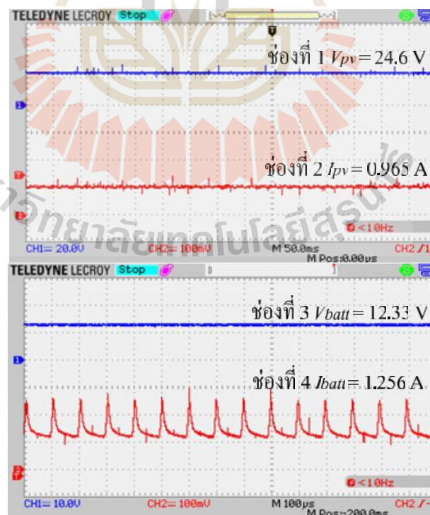
รูปที่ 5.21 ผลการทดสอบชุดทดสอบที่ความเข้มแสง 800 \text{ W/m}^2
