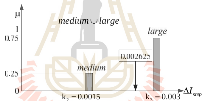
รูปที่ 5.14 ค่าเอต์พุตชัดเจนที่ได้จากการทำดีฟัซซี่ด้วยวิธีคำนวณน้ำหนักเฉลี่ย
