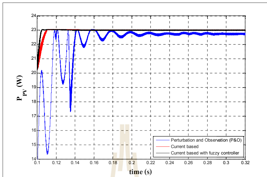
รูปที่ 6.2 พิจารณาเฉพาะช่วงที่ 1 ความเข้มแสง 600 \text{ W/m}^2 และอุณหภูมิ 25^\circ\text{C}
