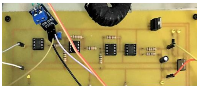
รูปที่ 4.19 วงจรตรวจจับกระแสที่ใช้งานจริง
