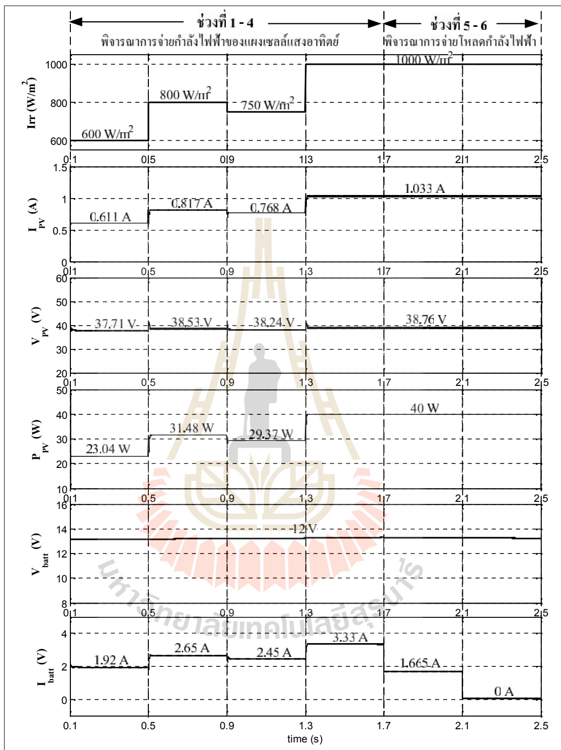
รูปที่ 5.15 ผลการจำลองสถานการณ์บนคอมพิวเตอร์ของวิธีอิงกระแสที่มีตัวควบคุมพีชชี
