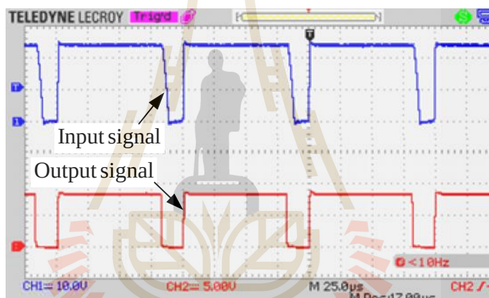
รูปที่ 4.39 ผลการทดสอบวงจรแยกโคดสัญญาณกรณีที่ 3 ค่าวัฏจักรหน้าที่ 80%
