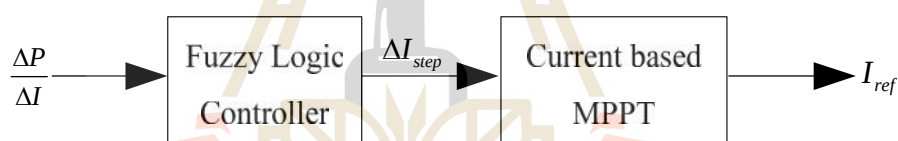
รูปที่ 5.8 ระบบควบคุมการหาค่า \Delta I_{step} สำหรับอัลกอริทึมในวิธีอิงกระแสโดยใช้ตัวควบคุมฟัซซี
