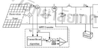
รูปที่ 6 ระบบการตามรอยจุดกำลังไฟฟ้าสูงสุดด้วยอัลกอริธึมอิงกระแส
