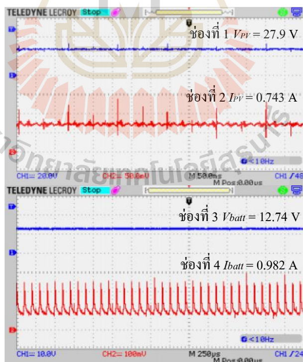
รูปที่ จ.3 เมื่อความเข้มแสงมีค่าเท่ากับ 600 \text{ W/m}^2
