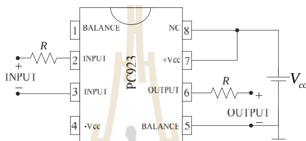
รูปที่ 4.36 วงจรแยกโคตสัญญาณที่ใช้ไอซี PC923
