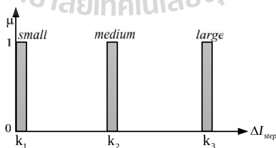
รูปที่ 5.10 ฟังก์ชันแสดงความเป็นสมาชิกของเอาต์พุต
