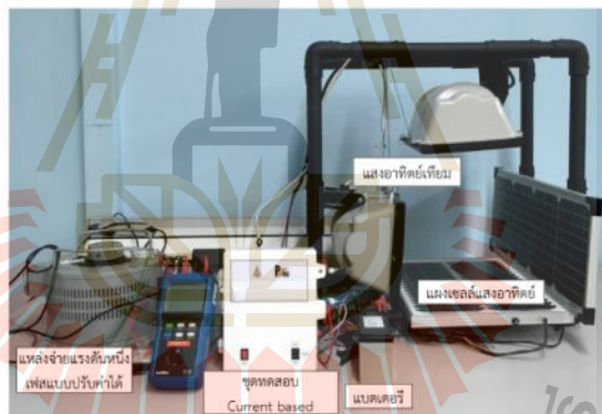
รูปที่ 16 ระบบฮาร์ดแวร์ชุดทดสอบการตามรอยจุดกำลังสูงสุดด้วยอัลกอริธึมอิงกระแส
