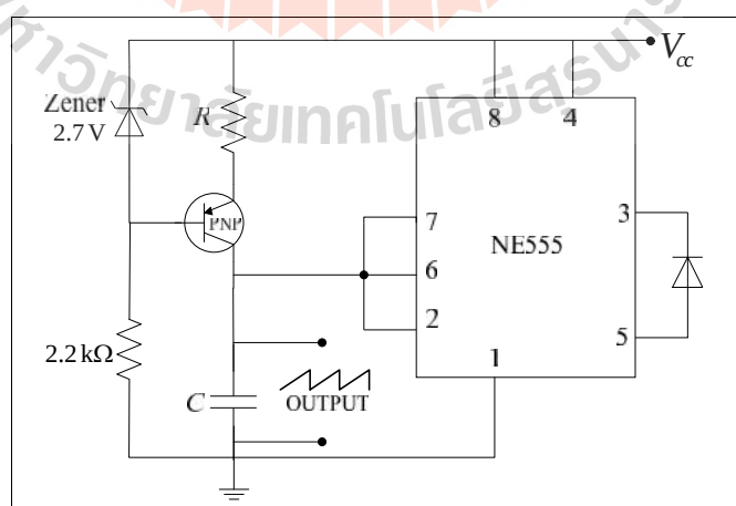
รูปที่ 4.26 วงจรสร้างสัญญาณฟันเลื่อย
