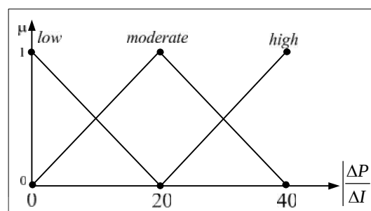
(ข) ฟังก์ชันแสดงความเป็นสมาชิกของอินพุต
