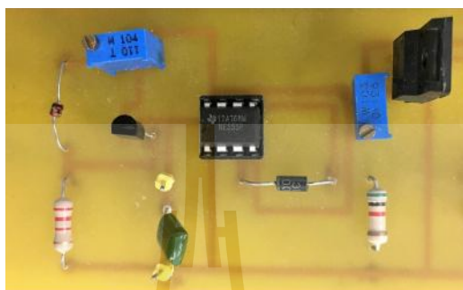
รูปที่ 4.28 วงจรสร้างสัญญาณฟันเลื่อยที่ใช้งานจริง
