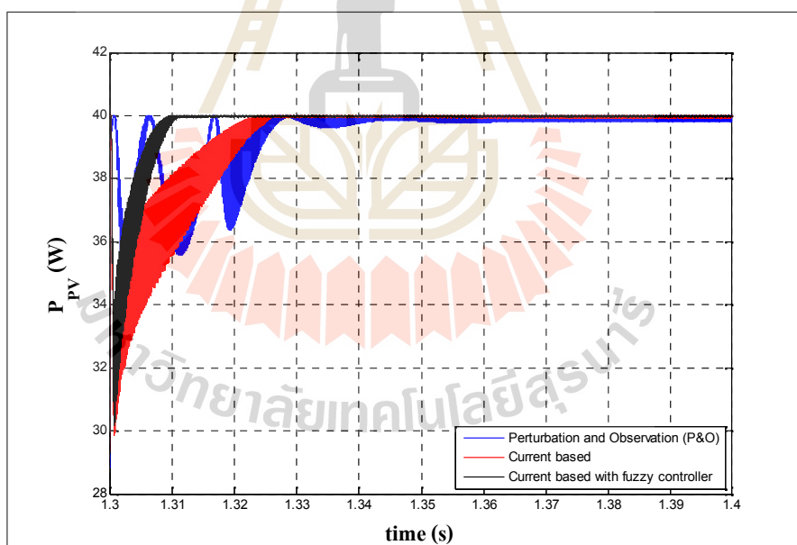
รูปที่ 6.5 พิจารณาเฉพาะช่วงที่ 4 ความเข้มแสง 1000 \text{ W/m}^2 และอุณหภูมิ 25^\circ\text{C}
