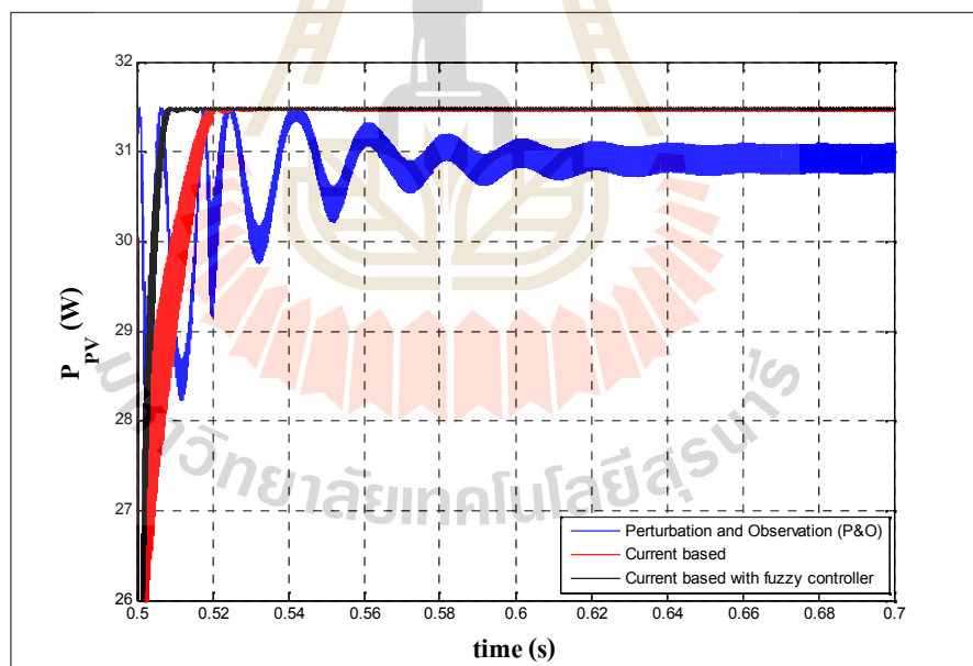
รูปที่ 6.3 พิจารณาเฉพาะช่วงที่ 2 ความเข้มแสง 800 \text{ W/m}^2 และอุณหภูมิ 25^\circ\text{C}
