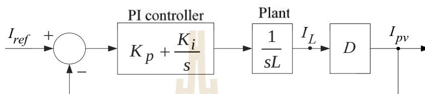
รูปที่ 4.22 ลูประแสไฟฟ้า
