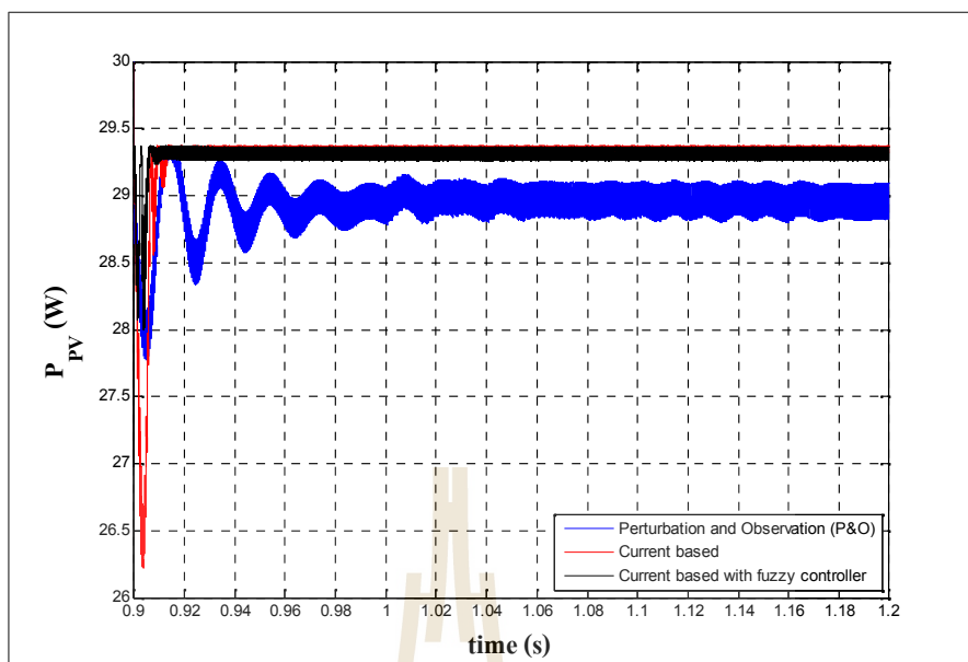
รูปที่ 6.4 พิจารณาเฉพาะช่วงที่ 3 ความเข้มแสง 750 \text{ W/m}^2 และอุณหภูมิ 25^\circ\text{C}
