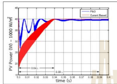
(ก) กำลังไฟฟ้าในสภาวะชั่วครู่ (transient)
