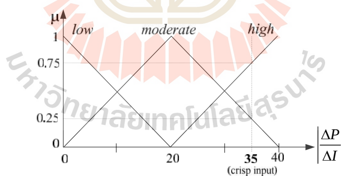
รูปที่ 5.12 การทำฟัซซีของระบบการตามรอยจุดกำลังสูงสุดด้วยวิธีอิงกระแสที่มีตัวควบคุมฟัซซี
