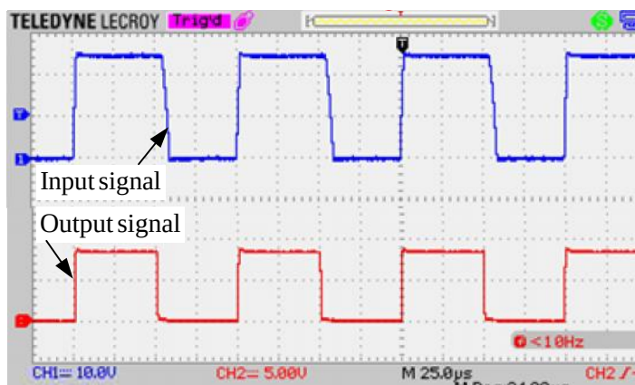
รูปที่ 4.38 ผลการทดสอบวงจรแยกโคดสัญญาณกรณีที่ 2 ค่าวัฏจักรหน้าที่ 50%
