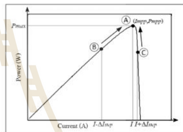
รูปที่ 7 คุณสมบัติเฉพาะกำลังและกระแสของเซลล์แสงอาทิตย์ สำหรับอัลกอริธึมอิงกระแส
