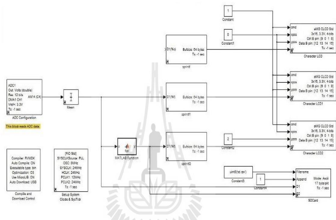
รูปที่ 3.5 แผนภาพโปรแกรม MATLAB แสดงเป็น simulink
