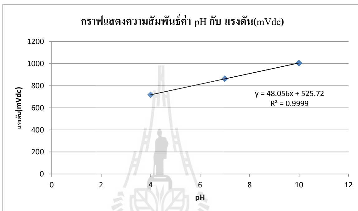
รูปที่ 4.4 กราฟแสดงความสัมพันธ์ของค่า pH ของบัฟเฟอร์มาตรฐานกับแรงดันที่วัดได้
