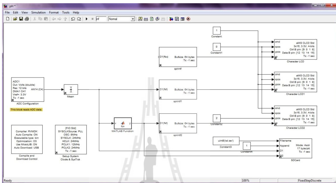
รูปที่ 4.12 แผนภาพโปรแกรม MATLAB SIMULINK ที่แสดงค่าแรงดันและค่า pH ผ่านบอร์ด Fio Std
