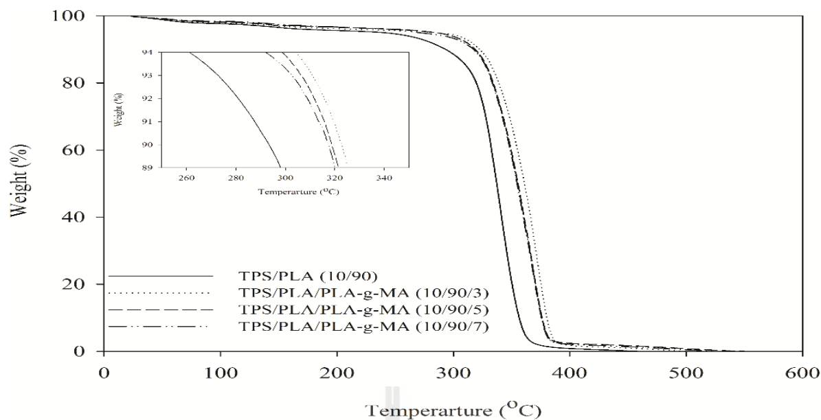
รูปที่ 4.20 กราฟ TGA พอลิเมอร์ผสมที่ไม่มีการปรับปรุงความเข้ากันได้ระหว่างเทอร์โมพลาสติกสตาร์ชกับพอลิแล็กติกแอซิดและพอลิเมอร์ผสมที่มีการปรับปรุงความเข้ากันได้ระหว่างเทอร์โมพลาสติกสตาร์ชกับพอลิแล็กติกแอซิดที่ปริมาณพอลิแล็กติกแอซิดกราฟมาเลือกแอนไฮดรายต่างๆ
