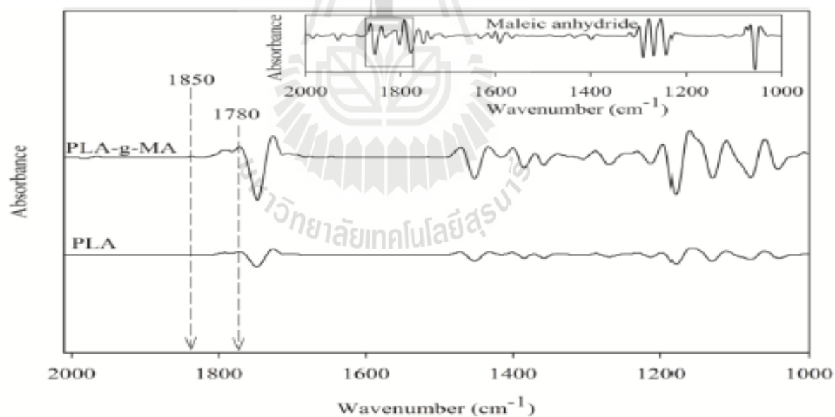
รูปที่ 4.2 อนุพันธ์อันดับสองของ FTIR สเปกตรัมของมาเลอิกแอนไฮไดร่า พอลิแลกติกแอซิด และพอลิแลกติกแอซิดกราฟมาเลอิกแอนไฮไดร่าที่ 1.0 เปอร์เซ็นต์โดยน้ำหนักของ 2,5-ไดเมทิล-2,5-ได-(เทอ-บิวทิเปอร์ออกไซด์)-เฮกเซน และ 5.0 เปอร์เซ็นต์โดยน้ำหนักของมาเลอิกแอนไฮไดร่า
