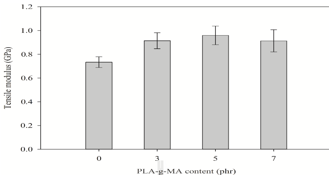
รูปที่ 4.15 มอดูลัสแรงดึงของพอลิเมอร์ผสมที่ไม่มีการปรับปรุงความเข้ากันได้ระหว่างเทอร์โมพลาสติกสตาร์ชกับพอลิแล็กติกแอซิด และพอลิเมอร์ผสมที่มีการปรับปรุงความเข้ากันได้ระหว่างเทอร์โมพลาสติกสตาร์ชกับพอลิแล็กติกแอซิดที่ปริมาณพอลิแล็กติกแอซิดกราฟมาเลอิกแอนไฮไดรต์ต่างๆ
