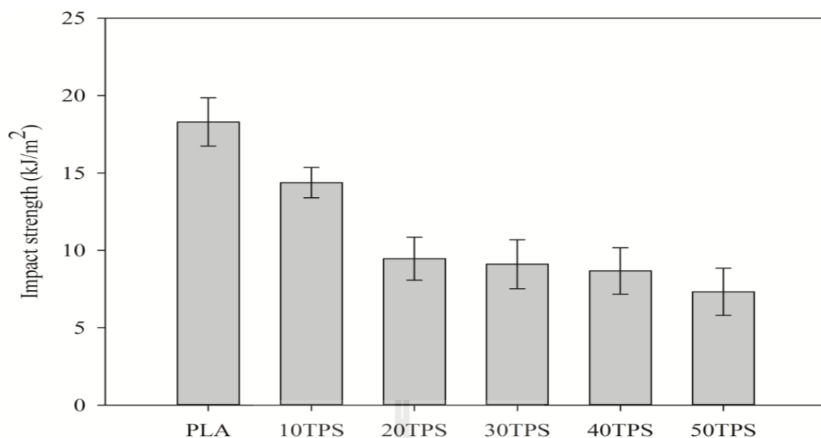
รูปที่ 4.7 ความต้านทานต่อแรงกระแทกของพอลิแลกติกแอซิด เทอร์โมพลาสติกสตา์ซ์ และพอลิเมอร์ผสมระหว่างเทอร์โมพลาสติกสตา์ซ์กับพอลิแลกติกแอซิดที่ปริมาณเทอร์โมพลาสติกสตา์ซ์ต่างๆ
