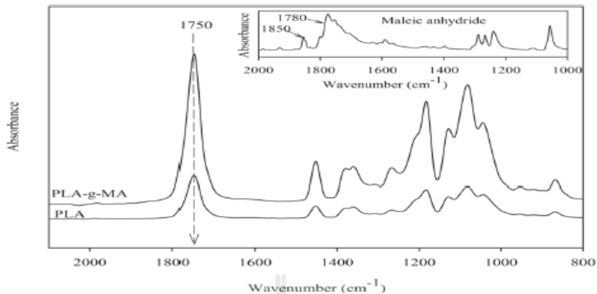
รูปที่ 4.1 FTIR สเปกตรัมของมาเลอิกแอนไฮไดร่า พอลิแลกติกแอซิด และพอลิแลกติกแอซิดกราฟมาเลอิกแอนไฮไดร่าที่ 1.0 เปอร์เซ็นต์โดยน้ำหนักของ 2,5-ไดเมทิล-2,5-ได-(เทอ-บิวทิเปอร์ออกไซด์)-เฮกเซน และ 5.0 เปอร์เซ็นต์โดยน้ำหนักของมาเลอิกแอนไฮไดร่า
