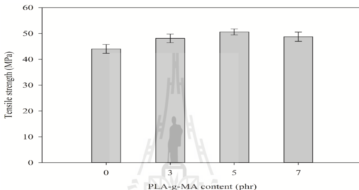
รูปที่ 4.14 ความต้านทานต่อแรงดึงของพอลิเมอร์ผสมที่ไม่มีการปรับปรุงความเข้ากันได้ระหว่างเทอร์โมพลาสติกสตา์ซกับพอลิแล็กติกแอซิด และพอลิเมอร์ผสมที่มีการปรับปรุงความเข้ากันได้ระหว่างเทอร์โมพลาสติกสตา์ซกับพอลิแล็กติกแอซิดที่ปริมาณพอลิแล็กติกแอซิดกราฟมาเลอิกแอนไฮไดรด์ต่างๆ
