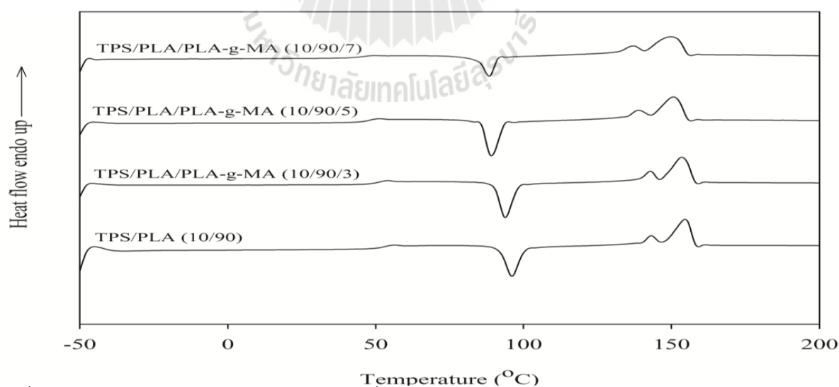
รูปที่ 4.19 กราฟ DSC ของพอลิเมอร์ผสมที่ไม่มีการปรับปรุงความเข้ากันได้ระหว่างเทอร์โมพลาสติกสตาร์ชกับพอลิแลกติกแอซิดและพอลิเมอร์ผสมที่มีการปรับปรุงความเข้ากันได้ระหว่างเทอร์โมพลาสติกสตาร์ชกับพอลิแลกติกแอซิดที่ปริมาณพอลิแลกติกแอซิดกราฟมาเลอิกแอนไฮไดรด์ต่างๆ (การให้ความร้อนครั้งที่ 2)
