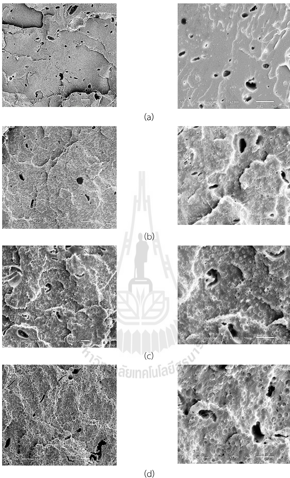
รูปที่ 4.26 ภาพถ่ายจากกล้องจุลทรรศน์อิเล็กตรอนแบบส่องกราดของพื้นผิวที่แตกหักในสถานะที่แช่แข็งที่กำลังขยาย 1000 เท่า (ซ้าย) และ 2000 เท่า (ขวา) ของ (a) TPS/PLA/PLA-g-MA (10/90/5phr) (b) TPS/PLA/PLA-g-MA/PBAT (9/81/5phr/10) (c) TPS/PLA/PLA-g-MA/PBAT (8/725phr/20) (d) TPS/PLA/PLA-g-MA/PBAT (7/63/5phr/30)
