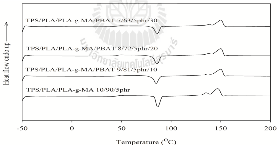
รูปที่ 4.28 กราฟ DSC ของพอลิเมอร์ผสมที่มีการปรับปรุงความเข้ากันได้ระหว่างเทอร์โมพลาสติกสตาร์ชกับพอลิแลกติกแอซิด และพอลิเมอร์ผสมที่มีการปรับปรุงความเข้ากันได้ระหว่างเทอร์โมพลาสติกสตาร์ช พอลิแลกติกแอซิดและพอลิบิวทีลีนอะดิเปรตโคเทอเรพทาเรตที่ปริมาณพอลิบิวทีลีนอะดิเปรตโคเทอเรพทาเรตต่างๆ (การให้ความร้อนครั้งที่ 2)
