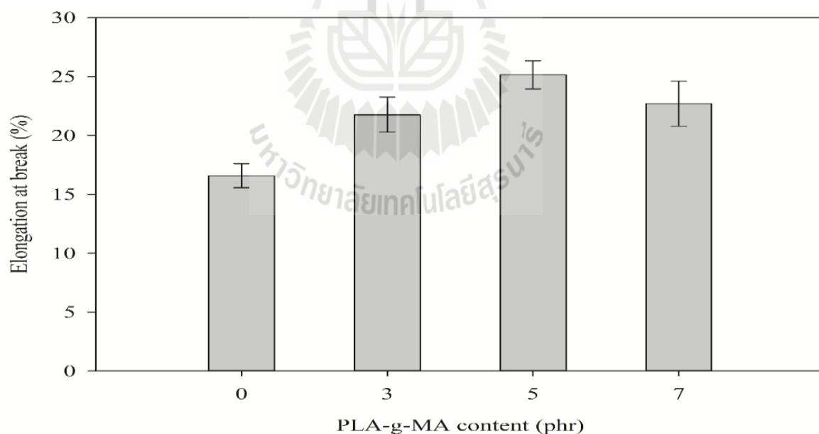
รูปที่ 4.16 ระยะยืด ณ จุดขาดของพอลิเมอร์ผสมที่ไม่มีการปรับปรุงความเข้ากันได้ระหว่างเทอร์โมพลาสติกสตาร์ชกับพอลิแล็กติกแอซิด และพอลิเมอร์ผสมที่มีการปรับปรุงความเข้ากันได้ระหว่างเทอร์โมพลาสติกสตาร์ชกับพอลิแล็กติกแอซิดที่ปริมาณพอลิแล็กติกแอซิดกราฟมาเลอิกแอนไฮไดรต์ต่างๆ
