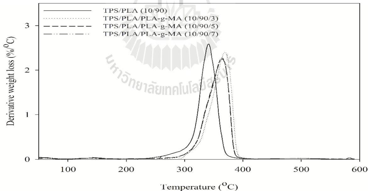
รูปที่ 4.21 กราฟ DTG ของพอลิเมอร์ผสมที่ไม่มีการปรับปรุงความเข้ากันได้ระหว่างเทอร์โมพลาสติกสตาร์ชกับพอลิแล็กติกแอซิดและพอลิเมอร์ผสมที่มีการปรับปรุงความเข้ากันได้ระหว่างเทอร์โมพลาสติกสตาร์ชกับพอลิแล็กติกแอซิดที่ปริมาณพอลิแล็กติกแอซิดกราฟมาเลือกแอนไฮดรายต่างๆ
