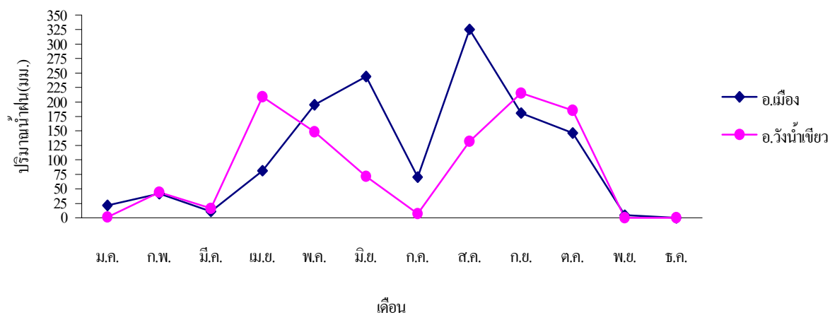
ภาพที่ 4.9 ปริมาณน้ำฝนประจำปี 2543 ของอำเภอเมือง และอำเภอวังน้ำเขียว จังหวัดนครราชสีมา
